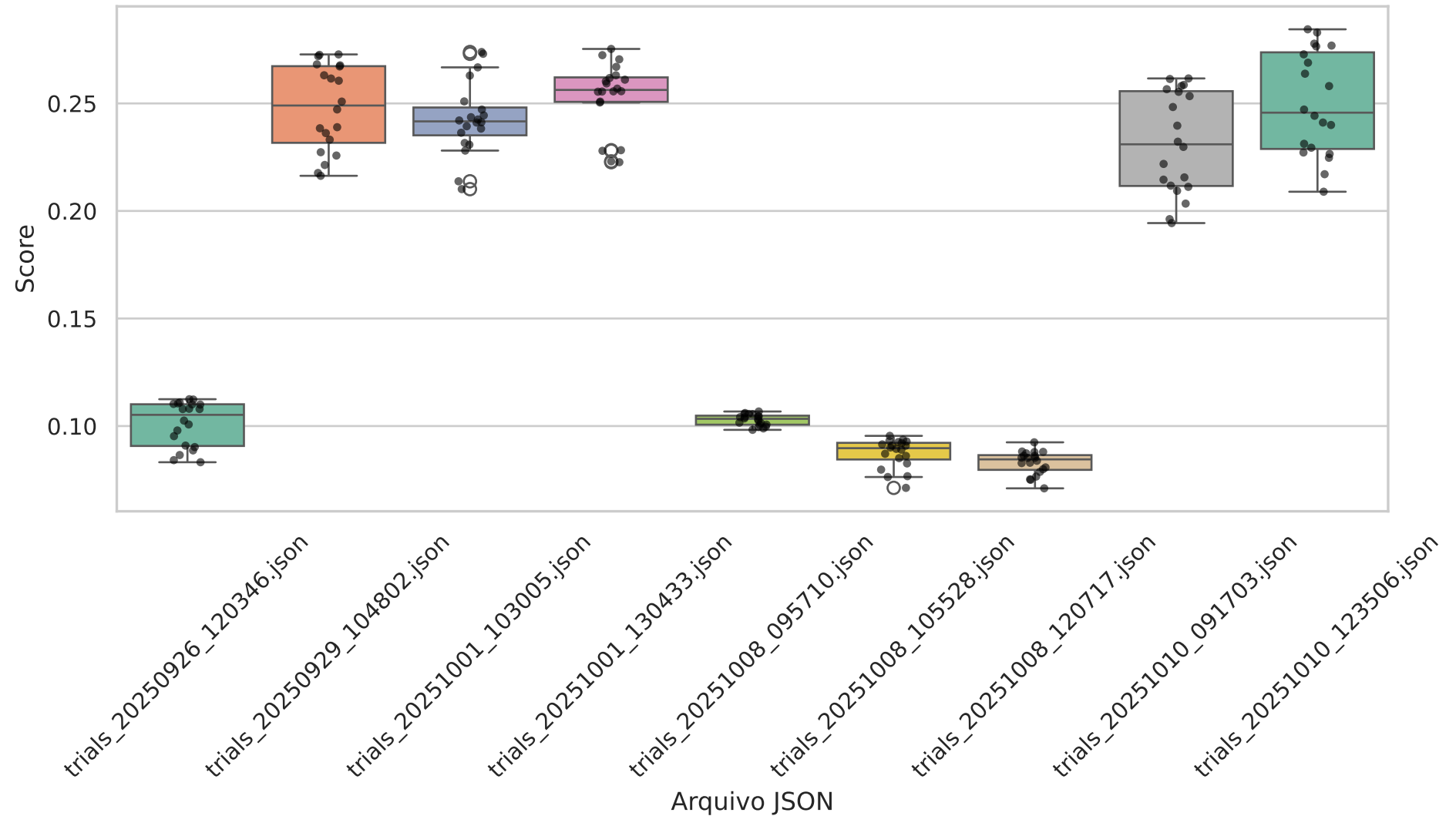
Distribuição dos Scores - Histogram Gradient Boosting
