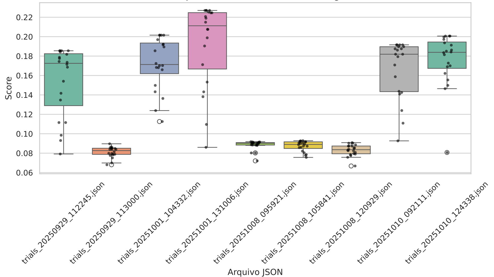
Distribuição dos Scores - K Nearest Neighbors
