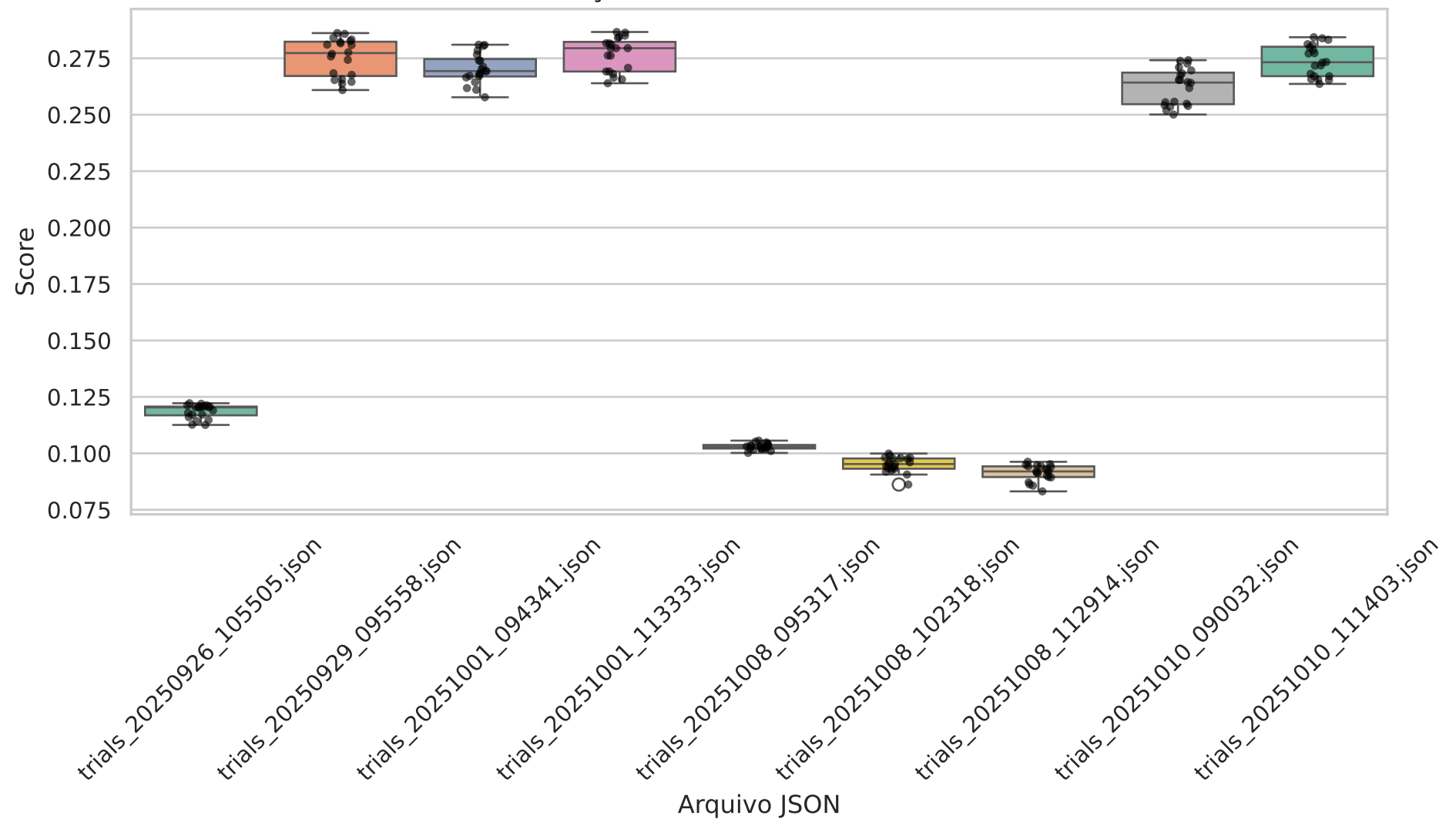
Distribuição dos Scores - Random Forest
