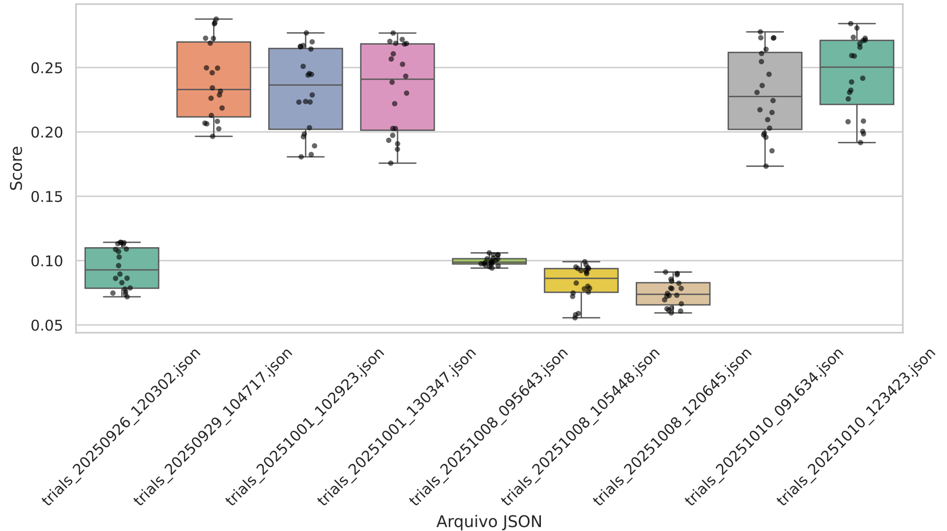
Distribuição dos Scores - Gradient Boosting
