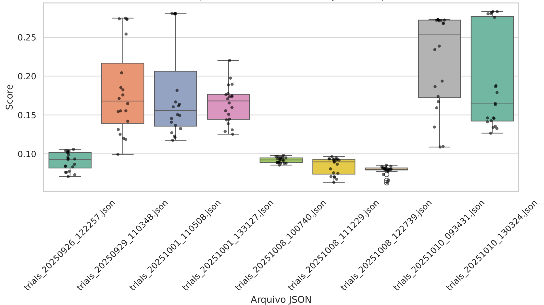
Distribuição dos Scores - Multi Layer Perceptron
