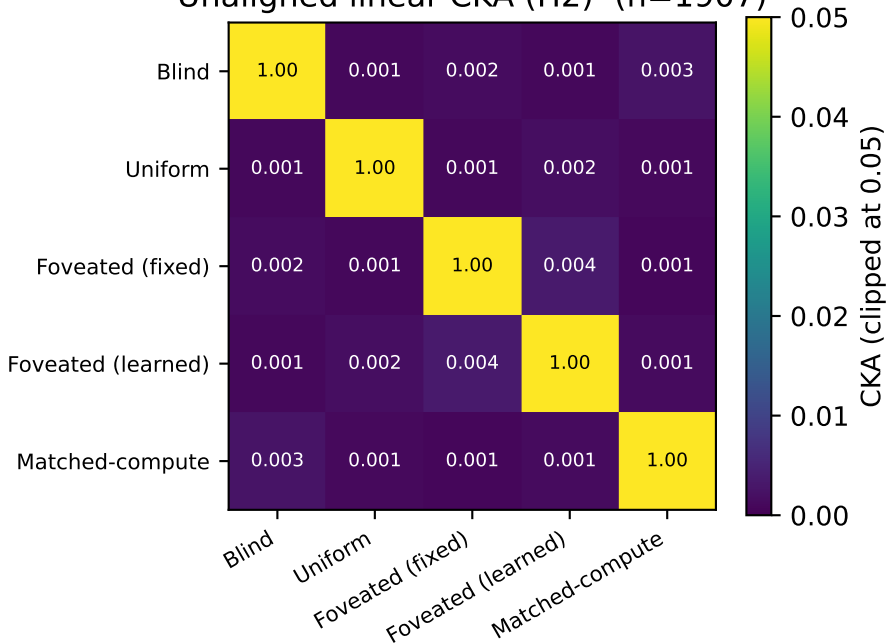
Unaligned linear CKA (H2) (n=1907)
