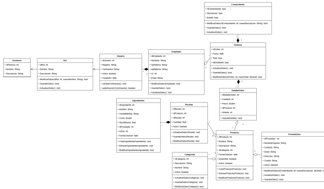
Diagrama 4: Diagrama de Clases del Sistema POS
