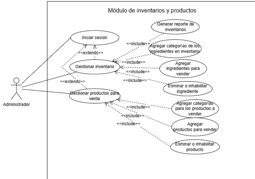
Diagrama 3: Diagrama de Casos de Uso del Sistema POS
