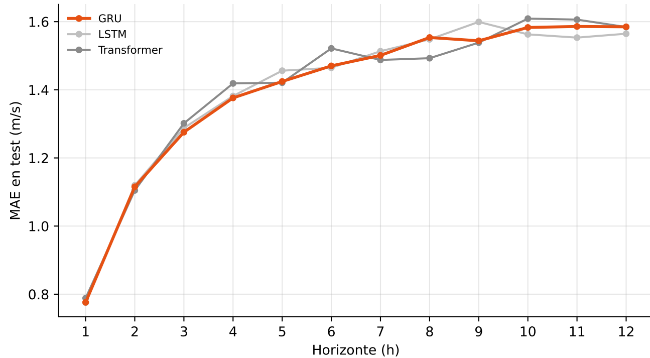
MAE por arquitectura y horizonte
