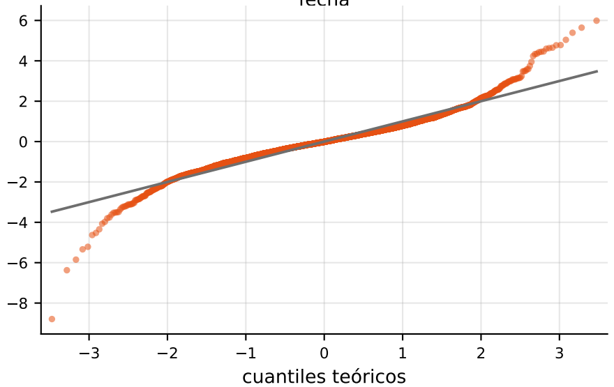
Gráfico Q-Q normal
