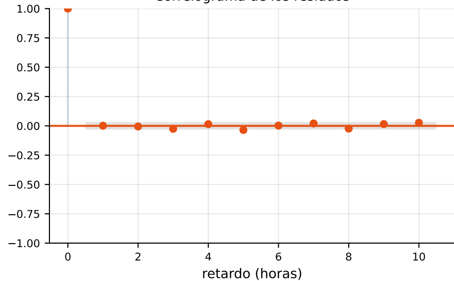
Correlograma de los residuos
