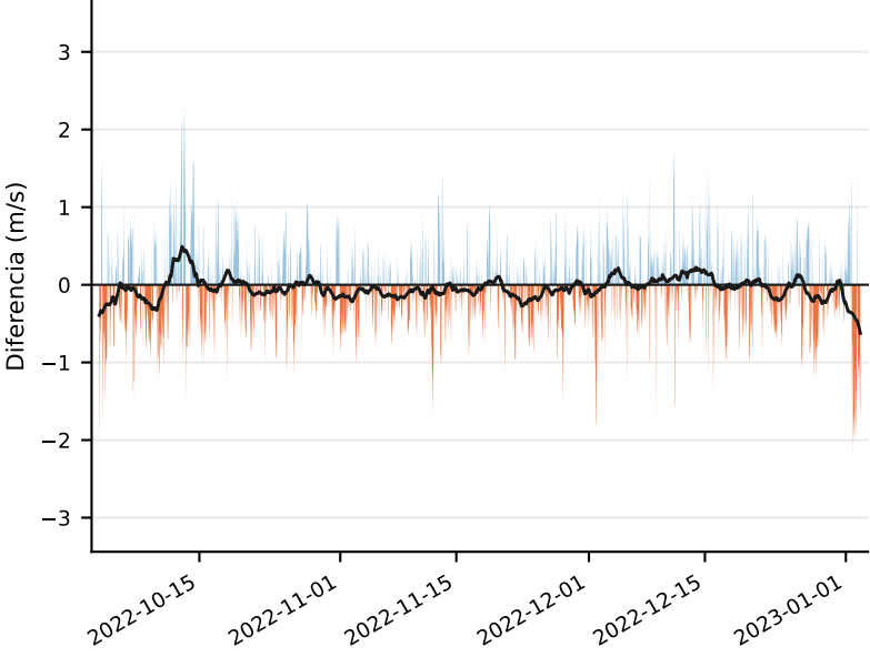
H = 10 h (media -0.047 m/s)
