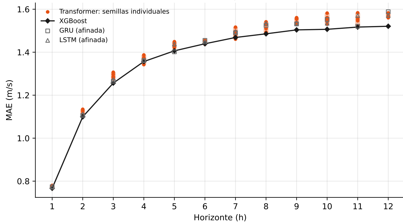
MAE de 5 semillas por horizonte
