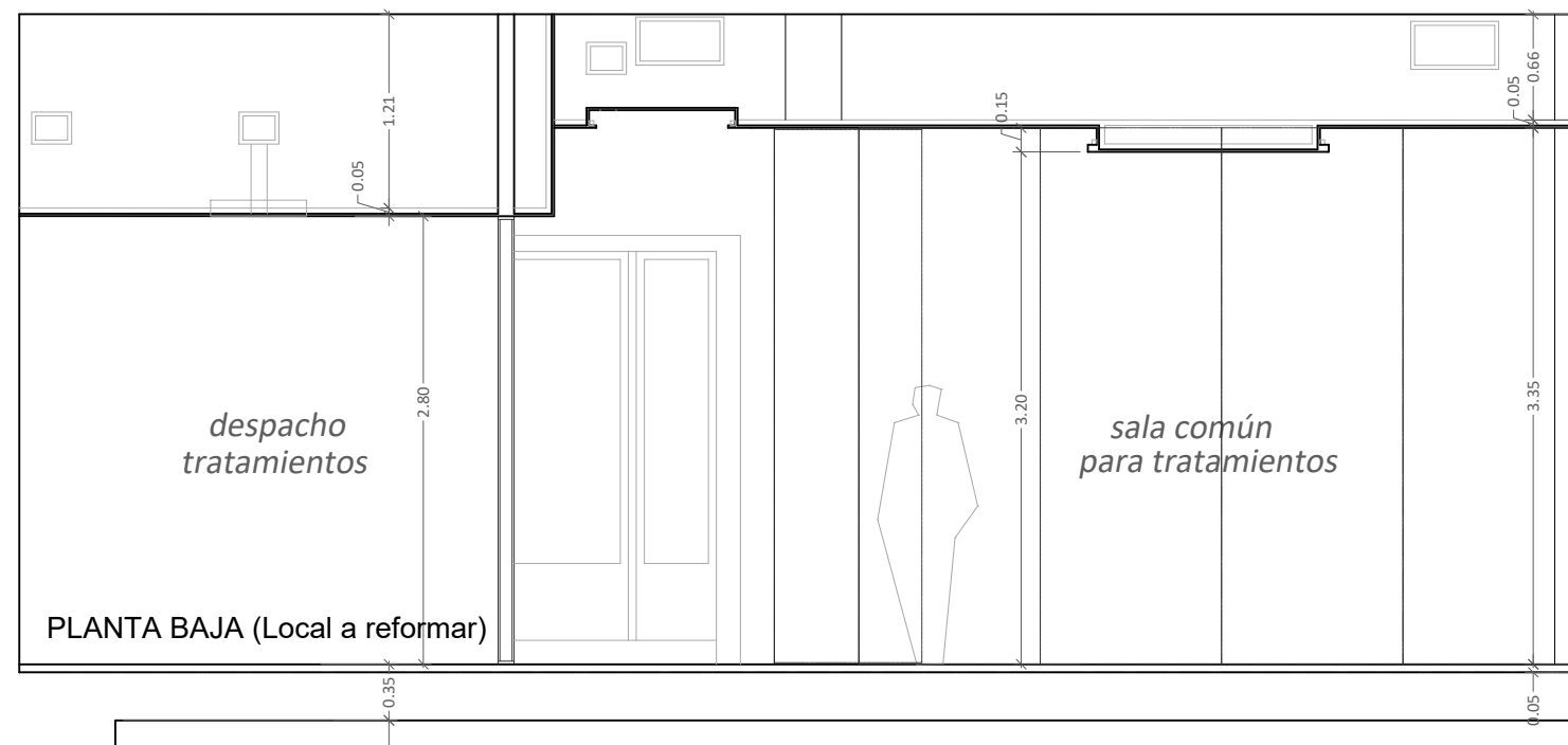
SECCIÓN B-B'
