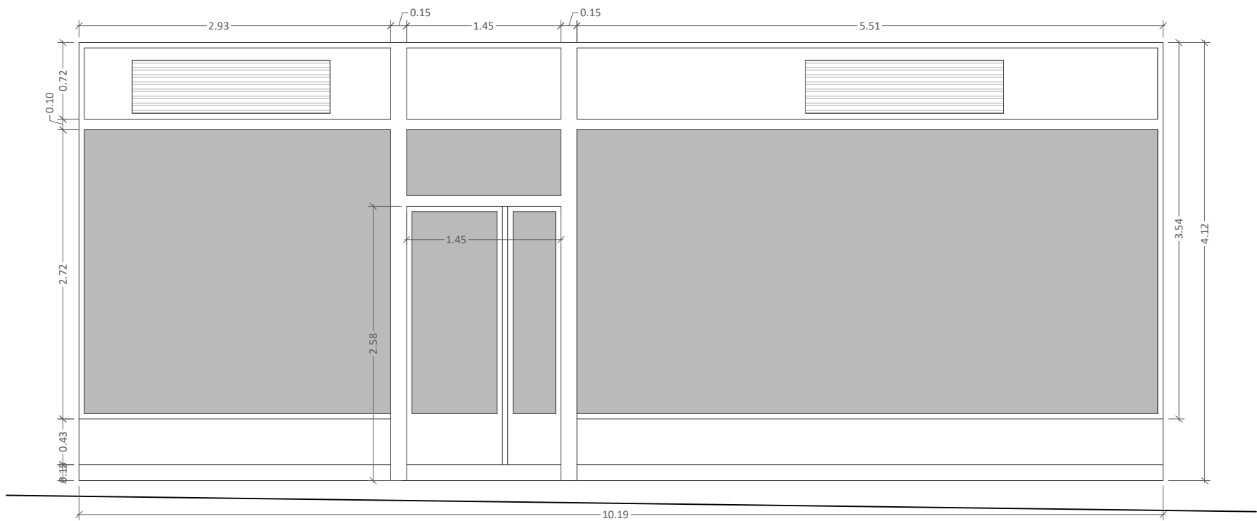
FACHADA PRINCIPAL (Oeste)
