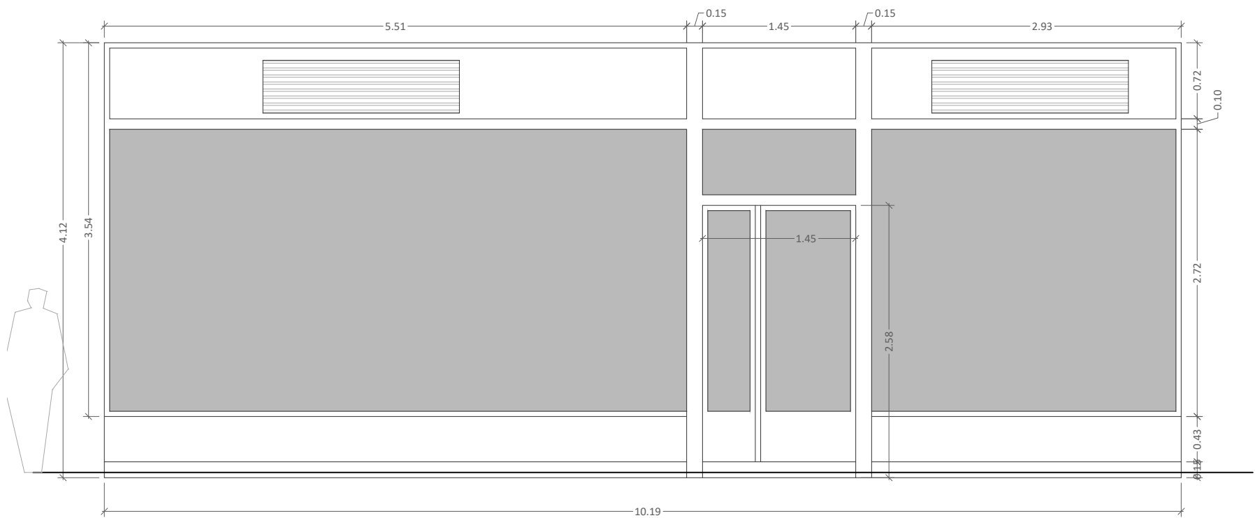
FACHADA TRASERA (Este)
