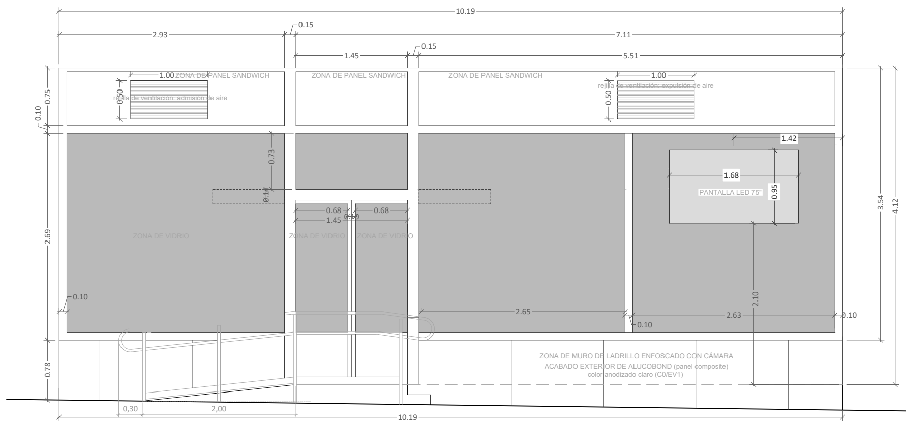
FACHADA PRINCIPAL (Oeste)
