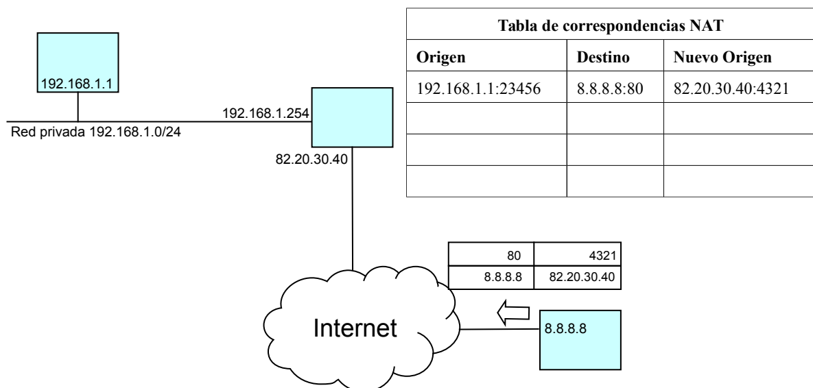
Figura 8: El servidor de Internet responde al origen del paquete
