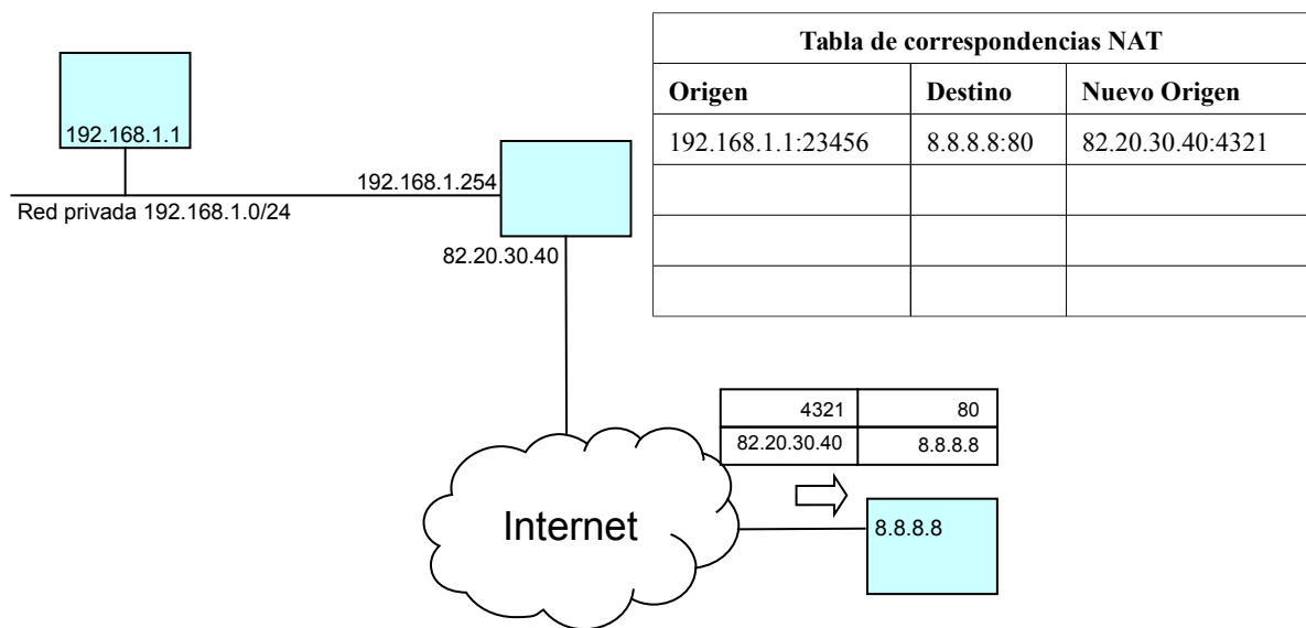
Figura 7: El paquete llega a su destino en Internet
