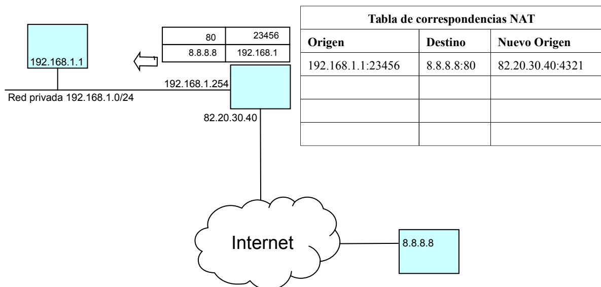
Figura 10: El router sabe que él no es el destino final, y deshace el cambio de direcciones
