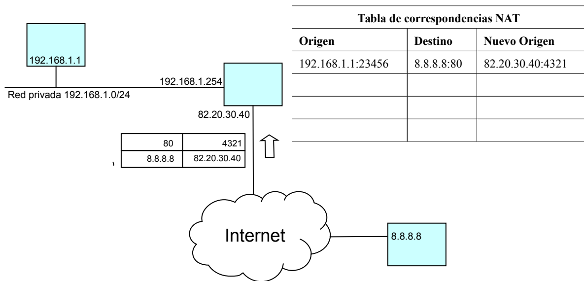
Figura 9: El paquete llega a la IP pública del router
