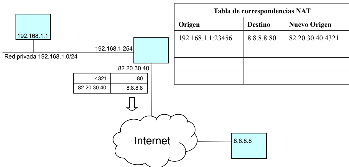
Figura 6: Lo envía sustituyendo la dirección IP de origen por la IP pública
