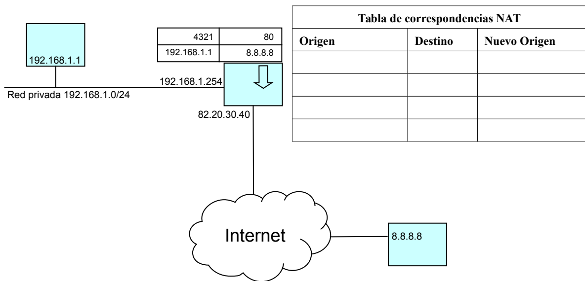
Figura 5: El router recibe el paquete
