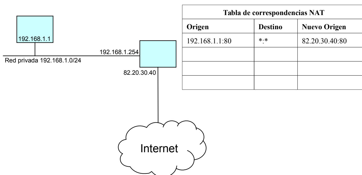
Figura 11: Servidor Web en 192.168.1.1 expuesto a Internet
