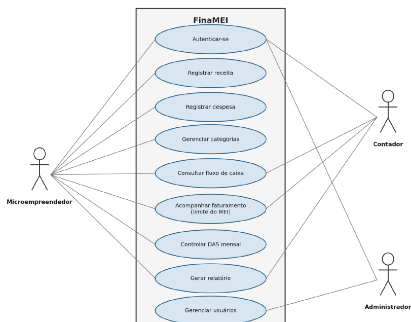
Figura – Diagrama de casos de uso do FinaMEI Fonte: elaborado pelos autores.
