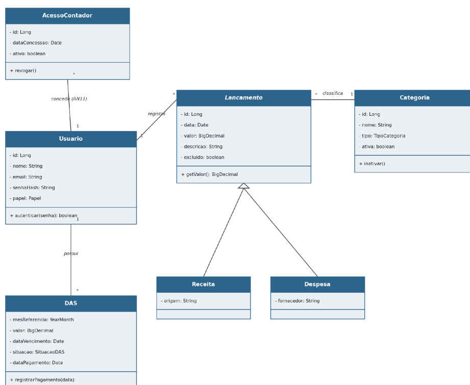
Figura – Diagrama de classes de domínio do FinaMEI Fonte: elaborado pelos autores.
