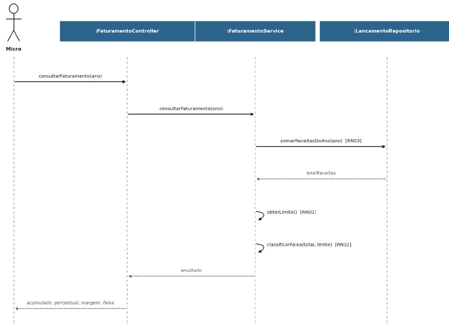
Figura – Diagrama de sequência de projeto – Consultar faturamento
