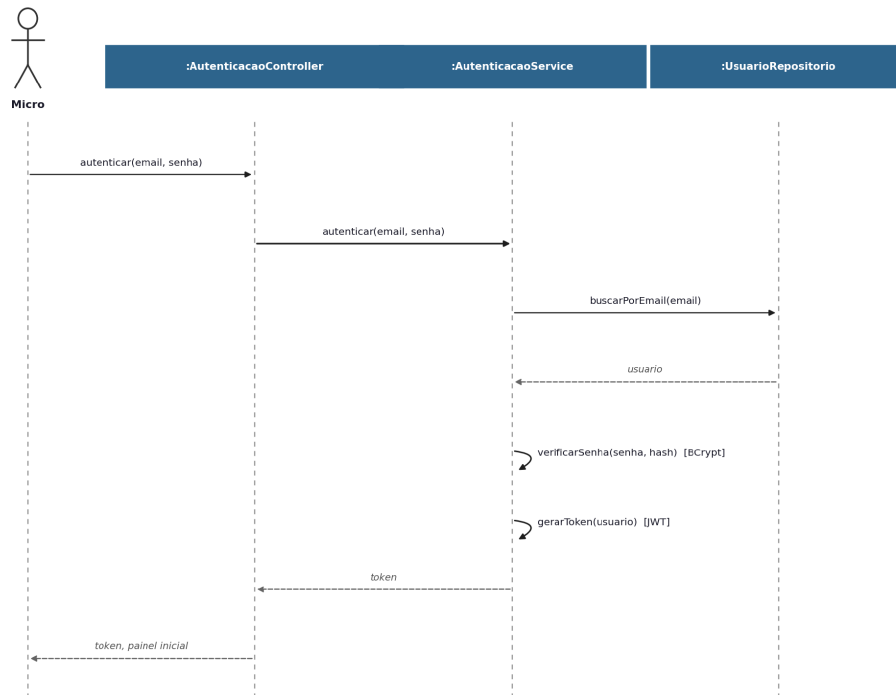
Figura – Diagrama de sequência de projeto – Autenticar-se Fonte: elaborado pelos autores.
