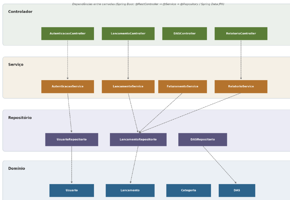
Figura – Arquitetura em camadas do FinaMEI Fonte: elaborado pelos autores.
