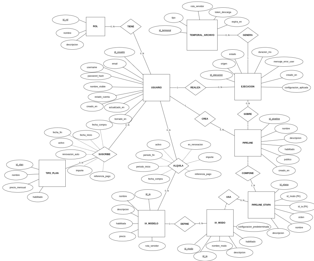
Figura C.1: Diagrama entidad-relación del sistema
