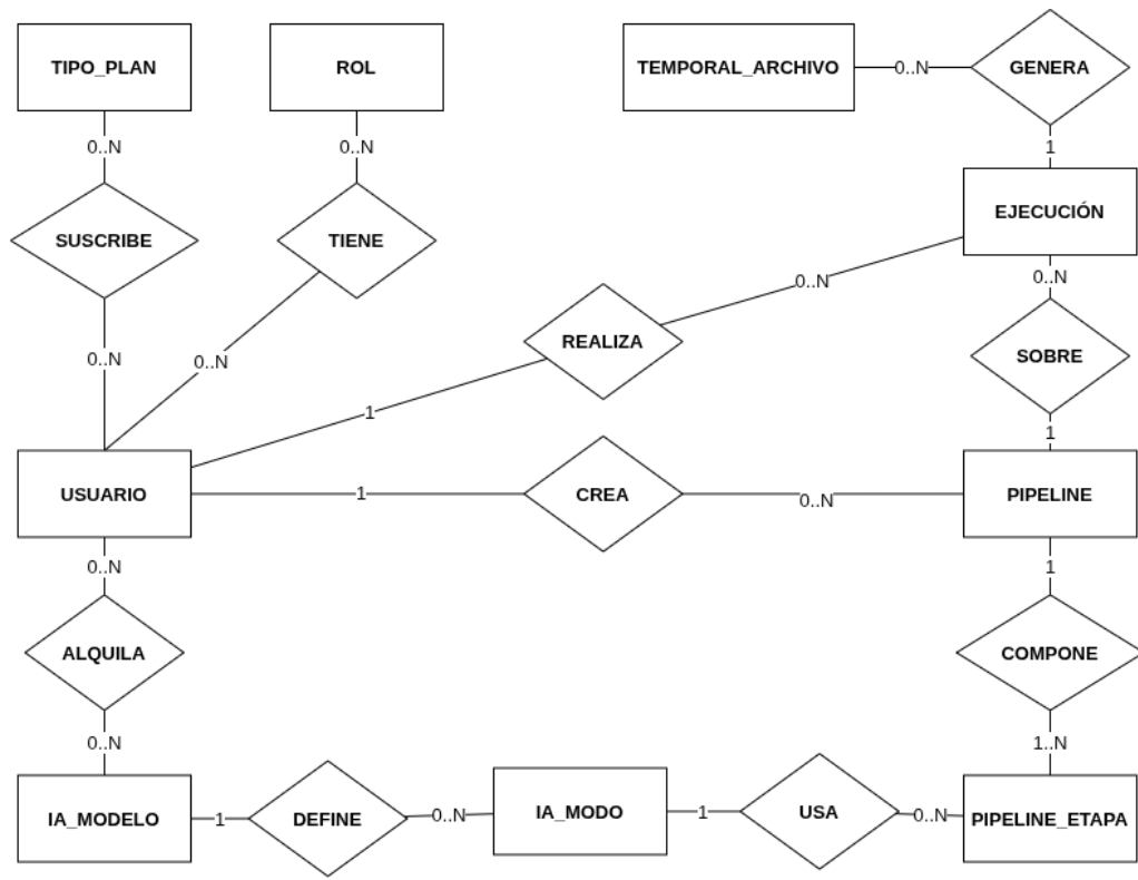
Figura C.1: Diagrama entidad-relación sin atributos del sistema.
