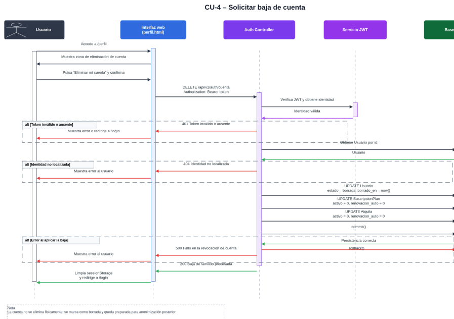
Figura C.9: Diagrama de secuencia del CU-4 Solicitar baja de cuenta.
