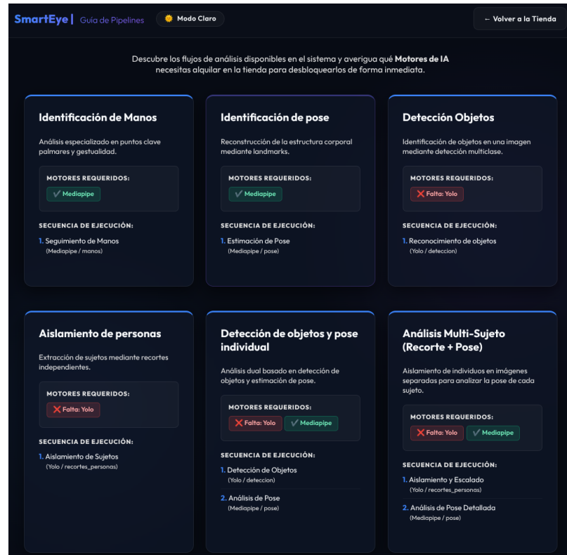
Figura E.10: Guía de pipelines disponibles y motores requeridos por cada flujo.
