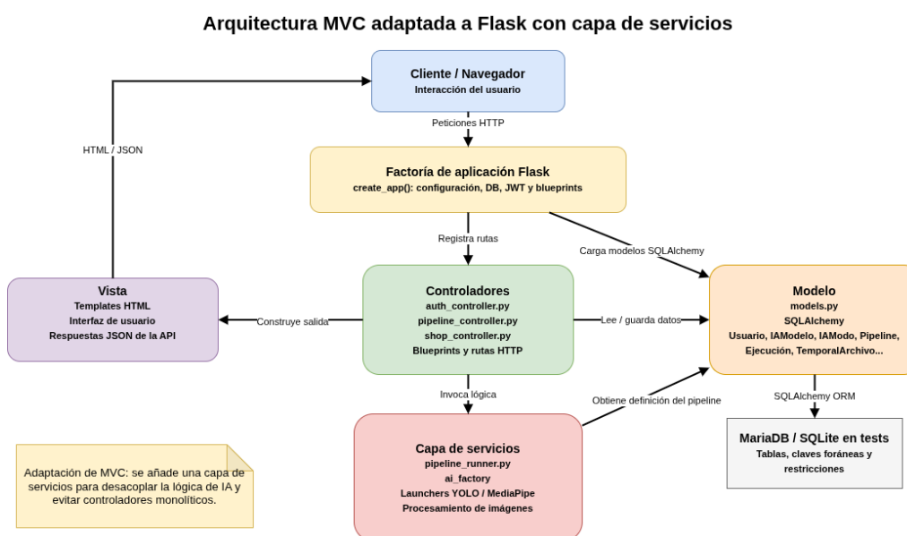
Figura C.3: Arquitectura MVC adaptada a Flask con capa de servicios.
