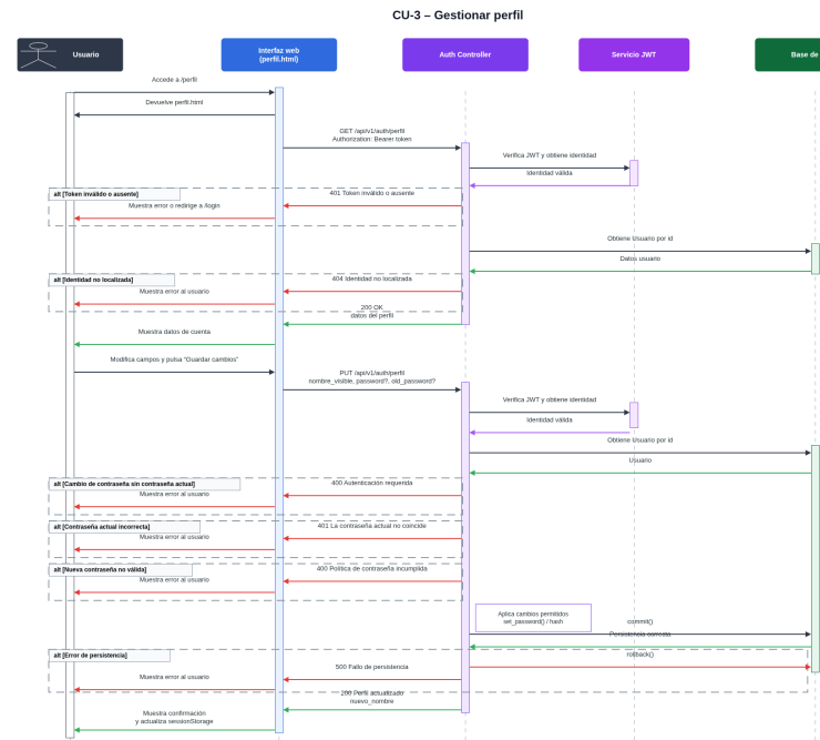
Figura C.8: Diagrama de secuencia del CU-3 Gestionar perfil.
