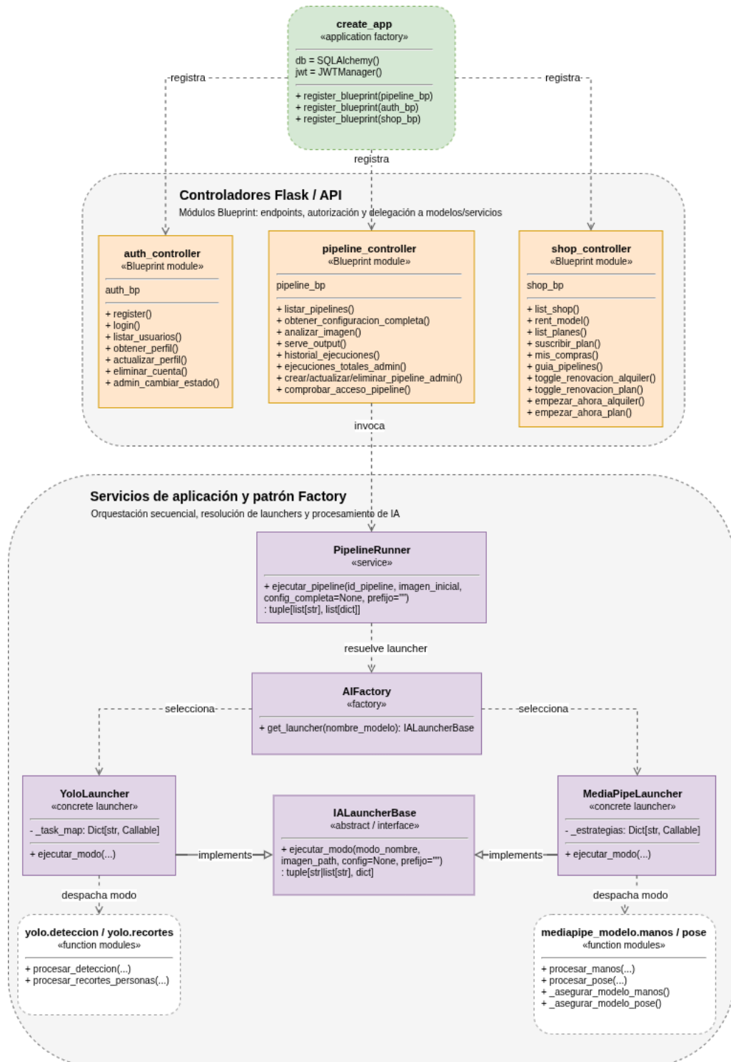
Figura C.5: Diagrama de clases y módulos principales de la capa de servicios.
