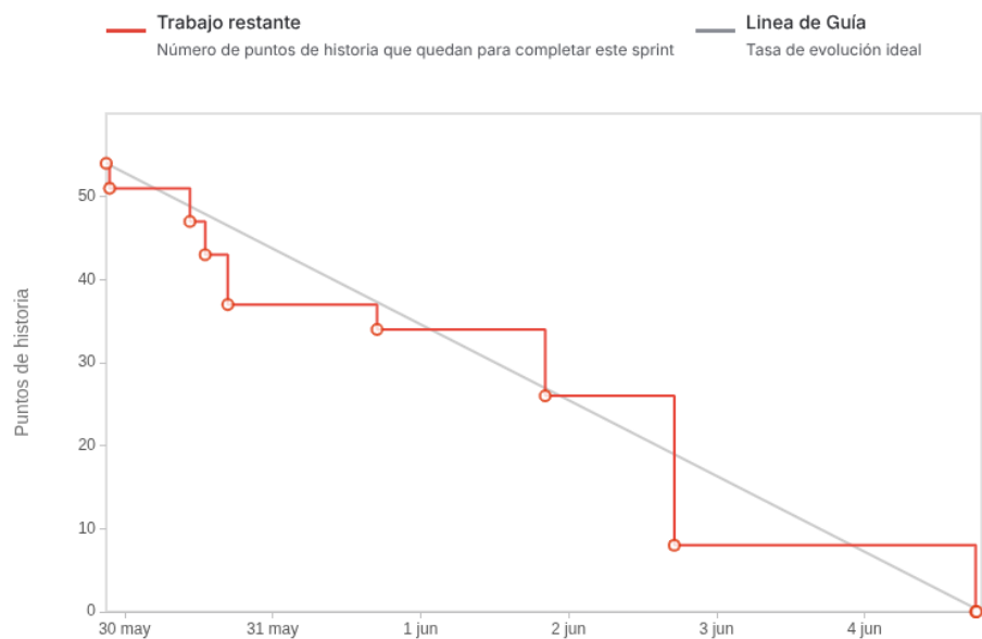
Figura A.16: Informe de trabajo completado del Sprint 16.
