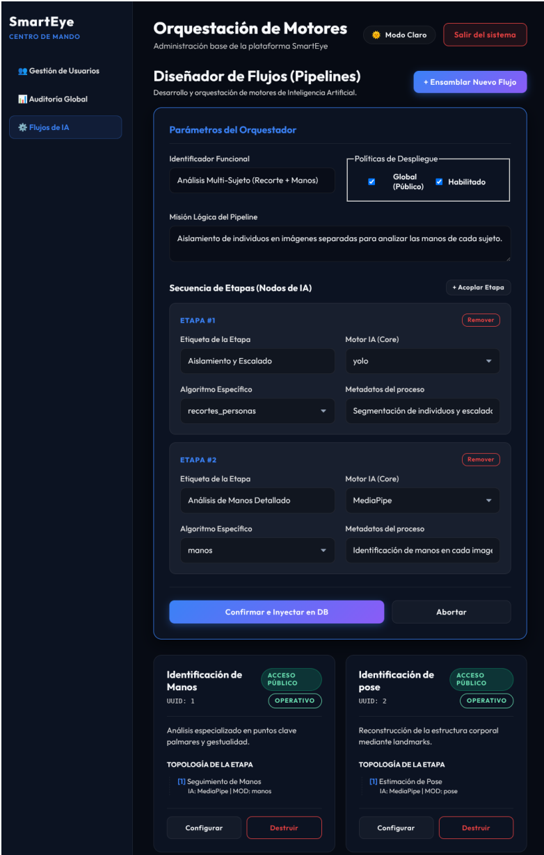
Figura E.15: Pantalla administrativa para diseñar y gestionar pipelines de IA.
