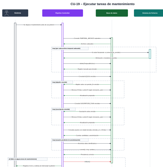
Figura C.24: Diagrama de secuencia del CU-19 Ejecutar tareas de mantenimiento.
