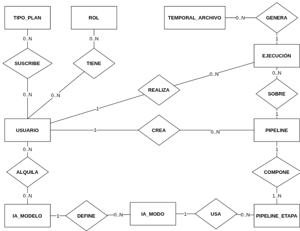
Figura C.1: Diagrama entidad-relación sin atributos del sistema.
