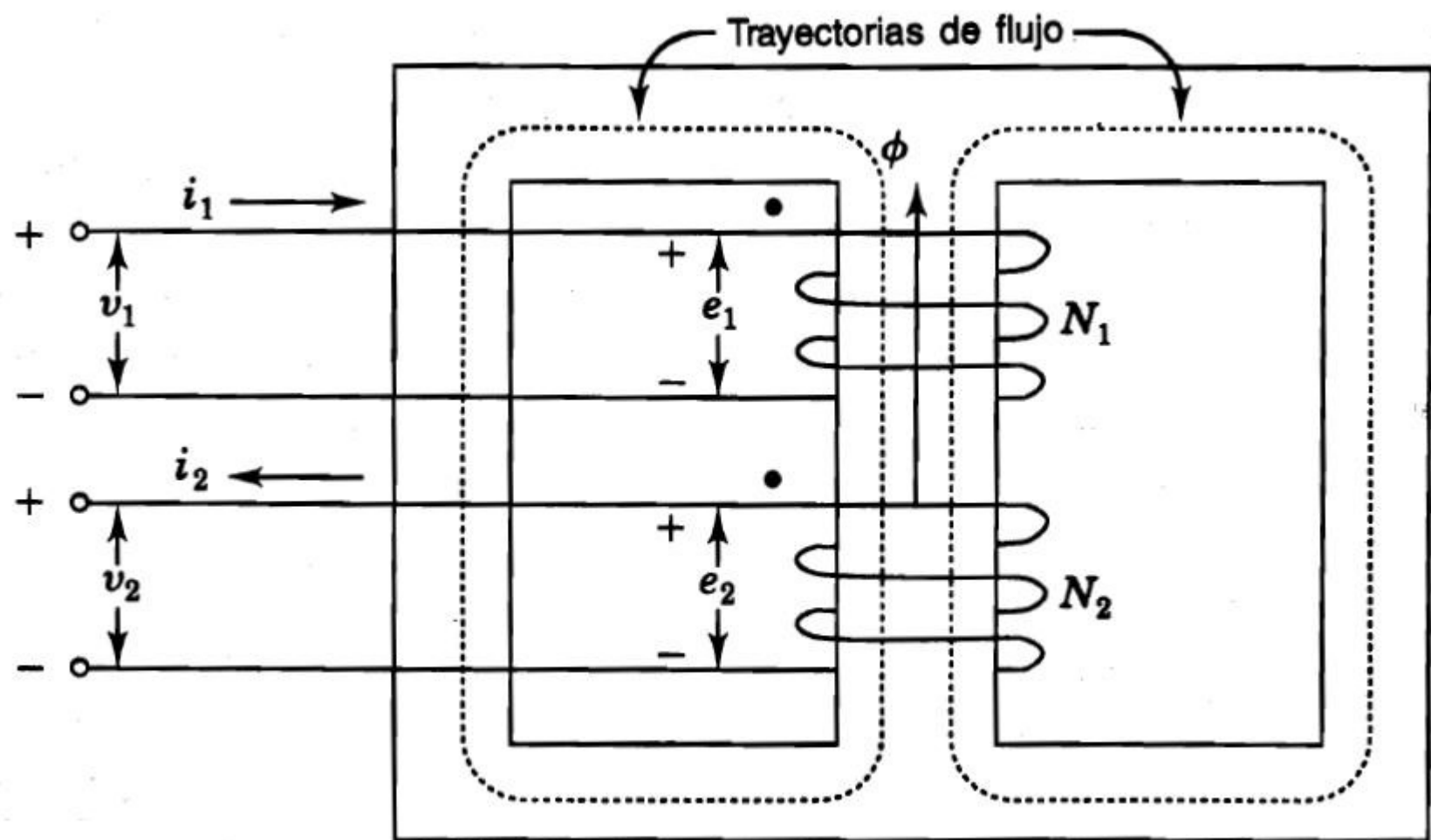
Transformador de dos devanados.
