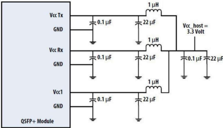
Figura 3: Filtro de Fonte de Alimentação Recomendado
