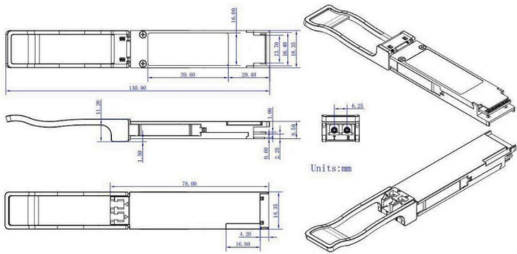
Figura 8: Desenho Técnico e Especificações Mecânicas
