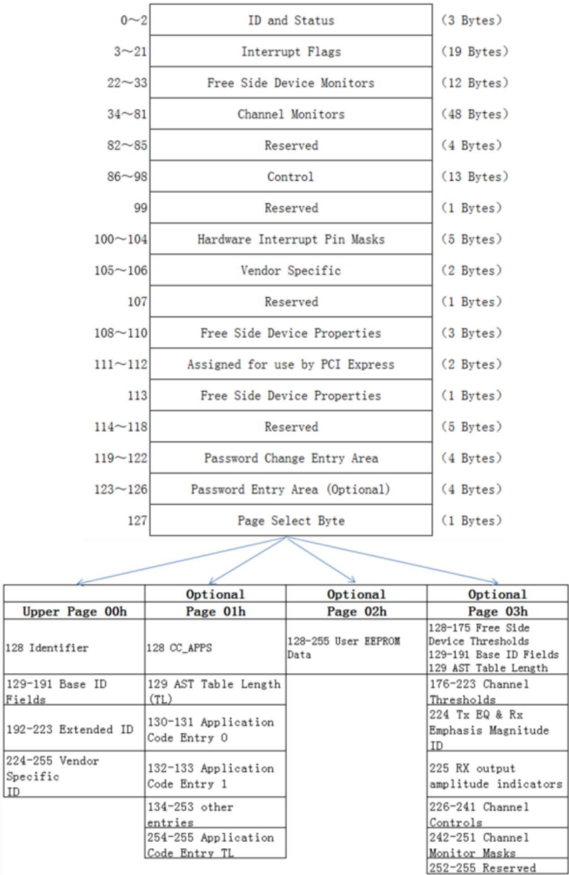
Figura 6: Mapa de Memória EEPROM
