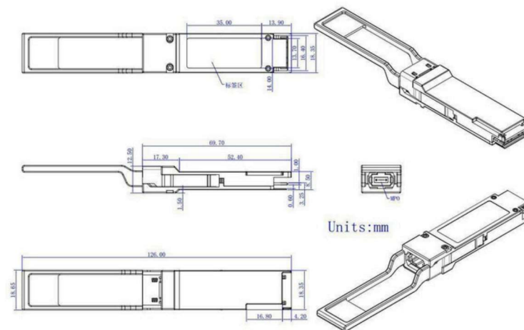
Figura 8: Desenho Técnico e Especificações Mecânicas
