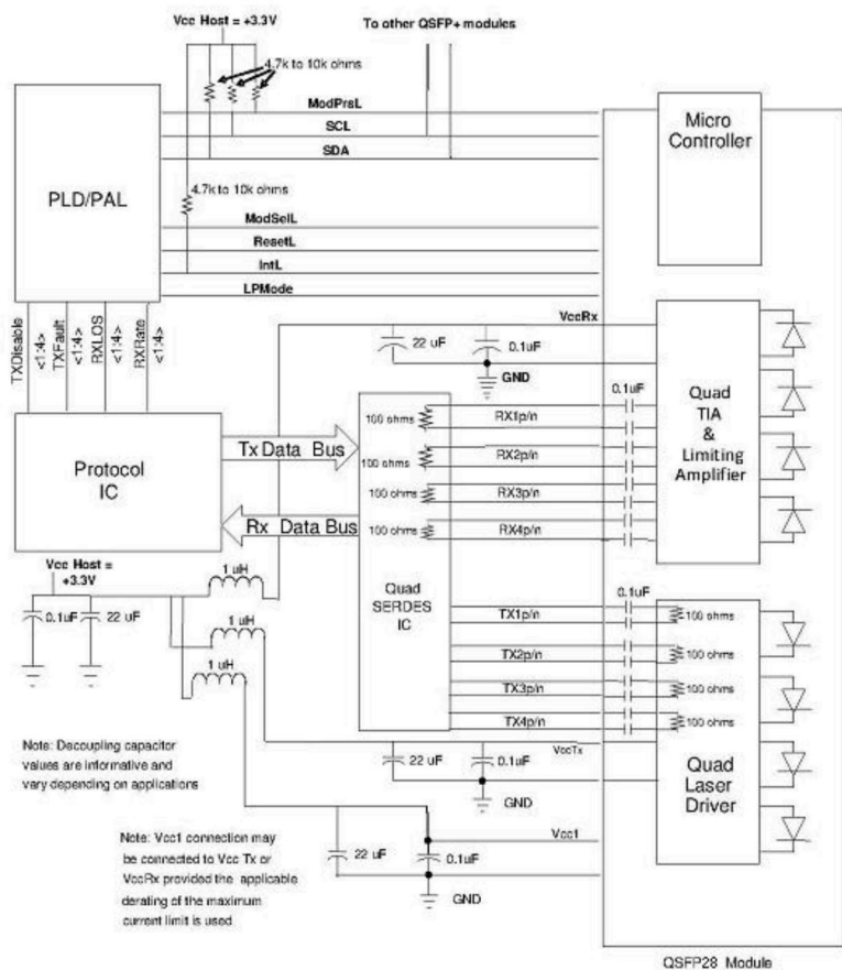
Figura 7: Esboço de Circuito Recomendado
