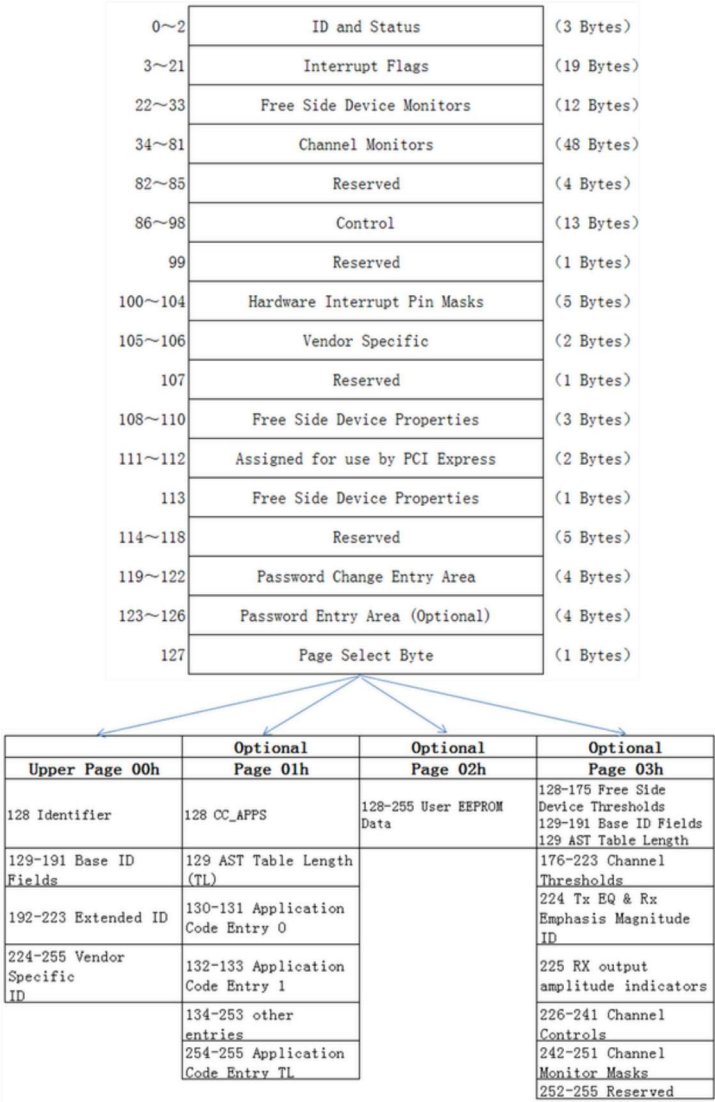
Figura 6: Mapa de Memória EEPROM
