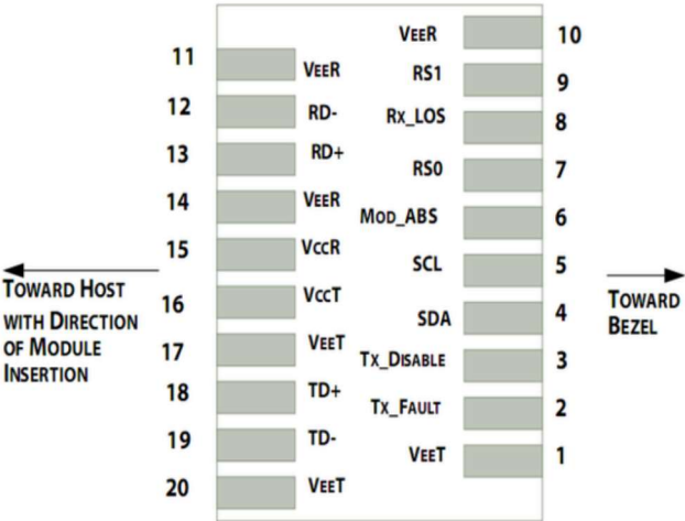
Figura 2: Pinagem do Bloco de Conectores na Placa Host
