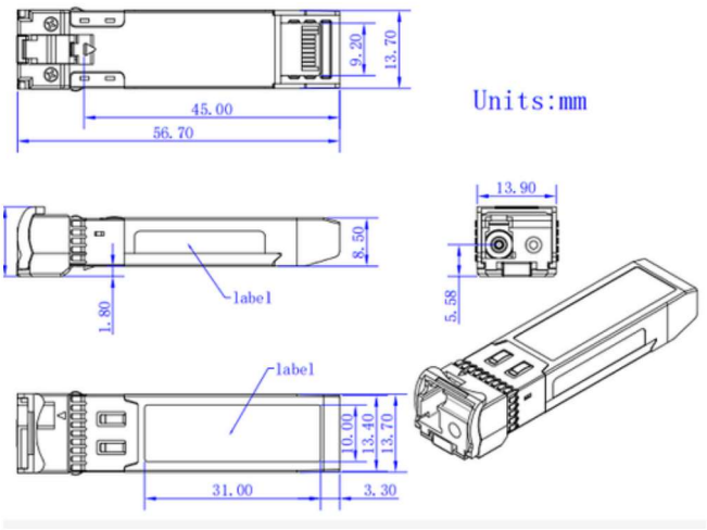
Figura 5: Desenho Técnico e Dimensões Mecânicas (em milímetros)
