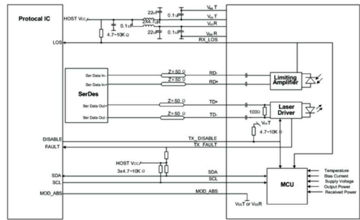
Figura 4: Esboço Recomendado do Circuito
