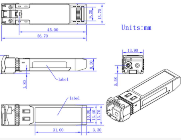
Figura 5: Desenho Técnico e Dimensões Mecânicas (em milímetros)
