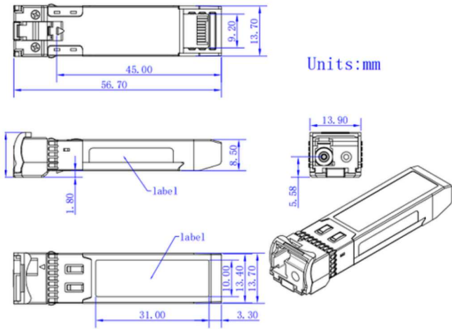
Figura 5: Desenho Técnico e Dimensões Mecânicas (em milímetros)
