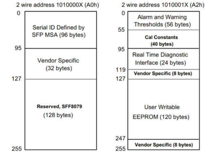
Figura 3: Mapa de Memória EEPROM
