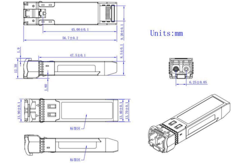
Figura 5: Desenho Técnico e Dimensões Mecânicas (em milímetros)
