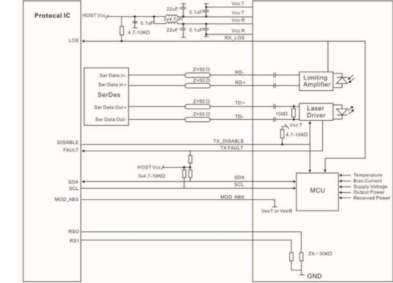
Figura 4: Esboço Recomendado do Circuito
