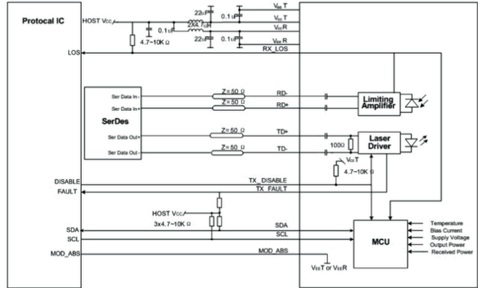
Figura 4: Esboço Recomendado do Circuito
