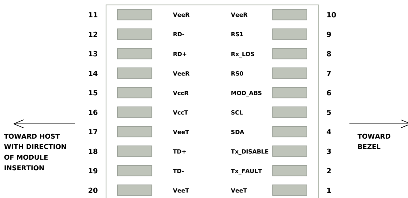
Pinagem do conector na placa host
