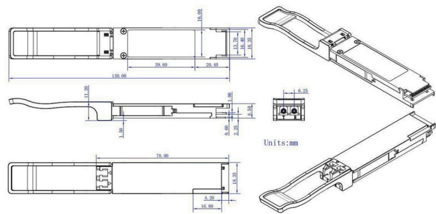
Figura 6: Desenho Técnico e Especificações Mecânicas (Unidades: mm)
