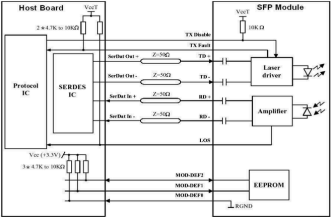
Figura 4: Esboço Recomendado do Circuito
