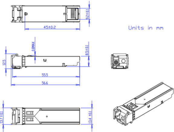
Figura 5: Desenho Técnico e Dimensões Mecânicas (em milímetros)
