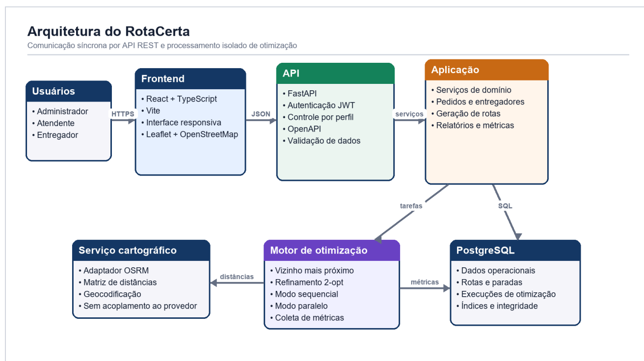
Figura 1 Arquitetura lógica e comunicação entre os componentes
