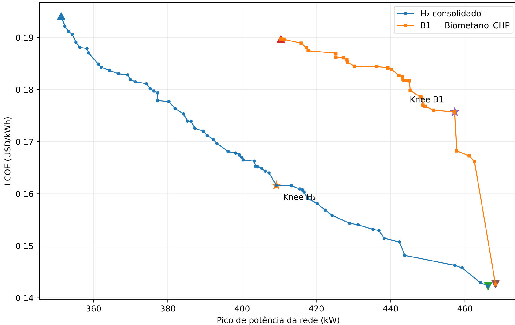
Fronteiras de Pareto consolidadas — H 2 × Biometano-CHP
