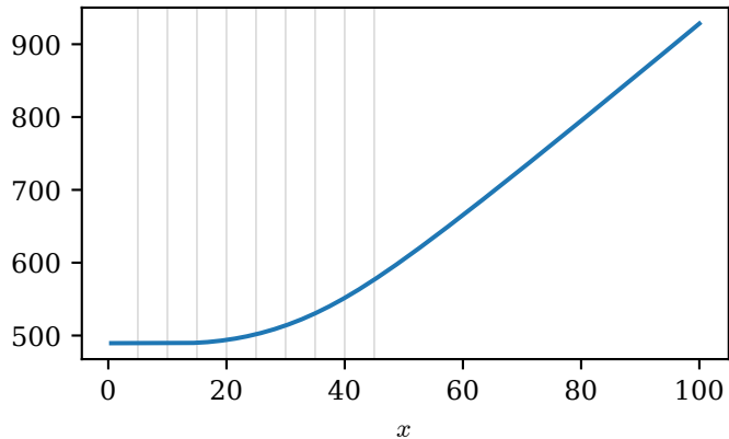
V(x)
