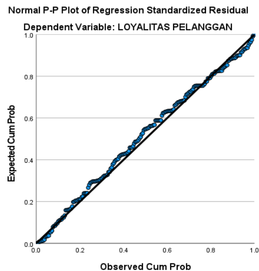
Gambar 2. Uji Normalitas (P-P plot)
