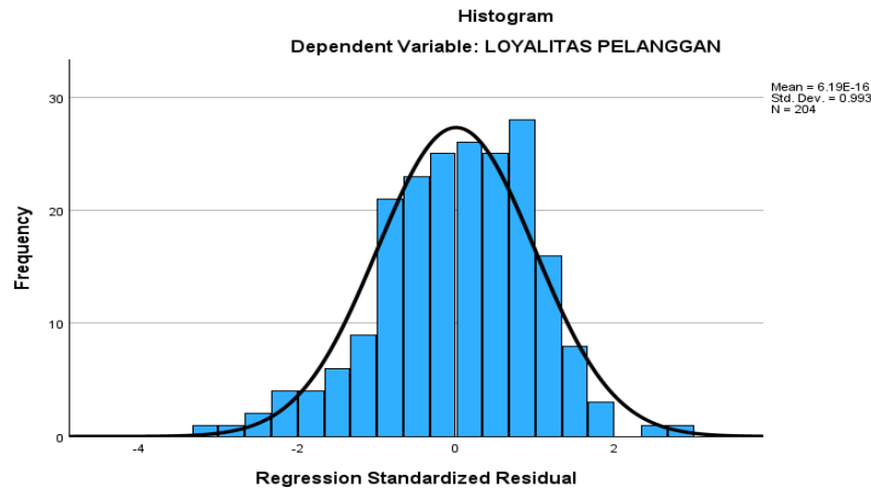
Gambar 3. Uji Normalitas (Histogram)
