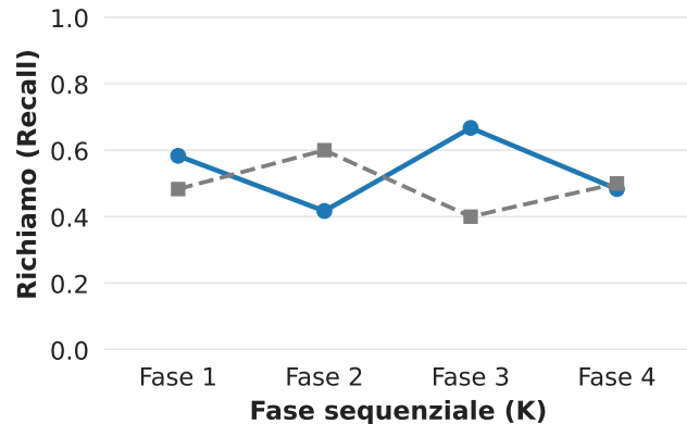
Richiamo (Recall)
