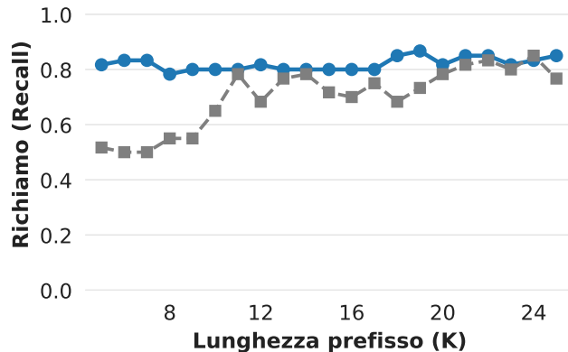
Richiamo (Recall)
