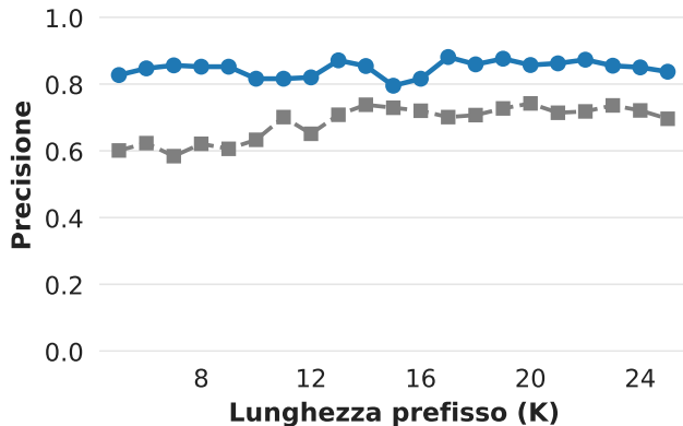
Precisione
