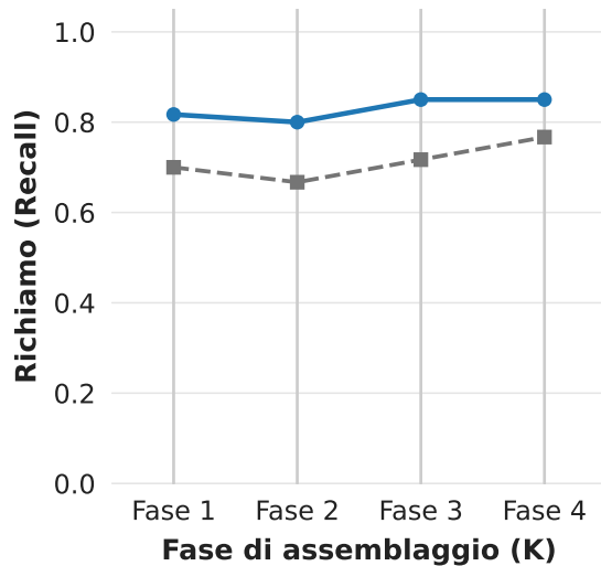
Richiamo (Recall)
