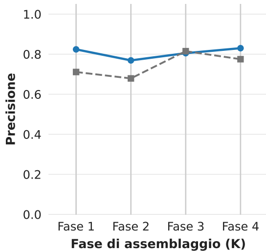
Precisione
