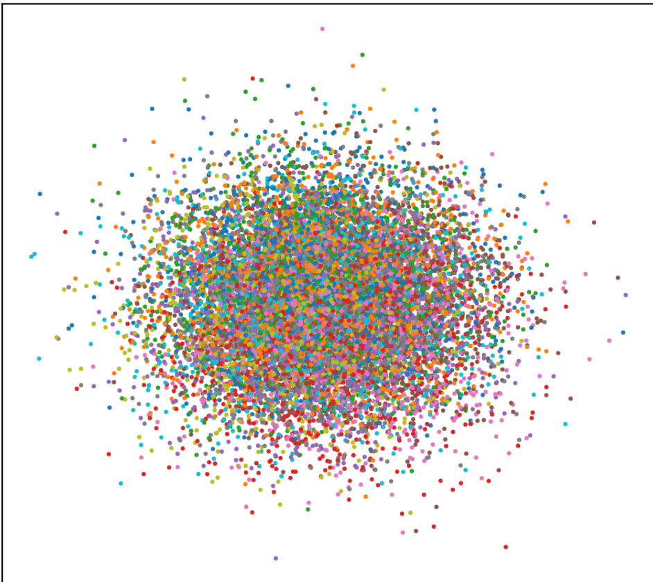
L2/Cosine — PCA
