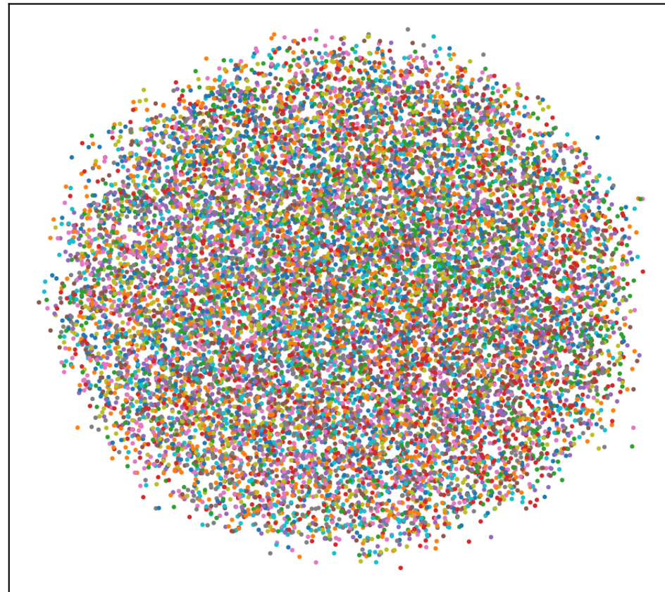
L2/Cosine — UMAP
