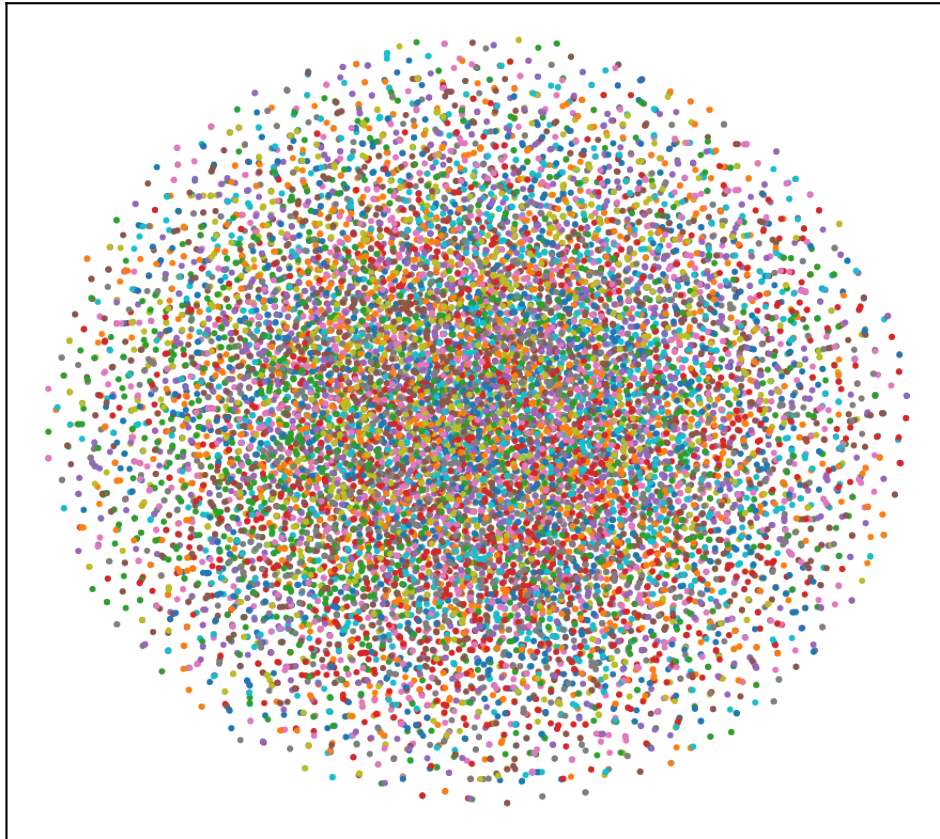
LayerNorm — t-SNE
