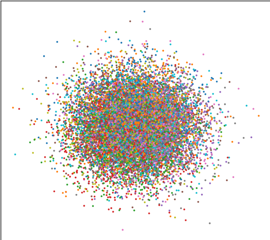
LayerNorm — PCA
