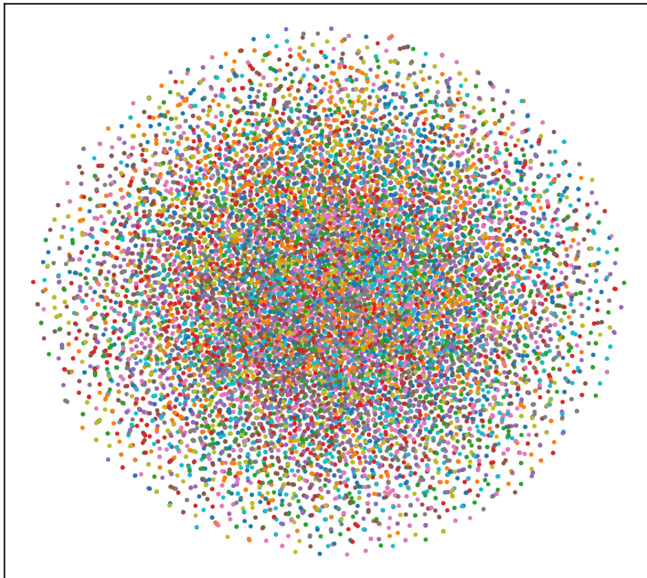
L2/Cosine — t-SNE
