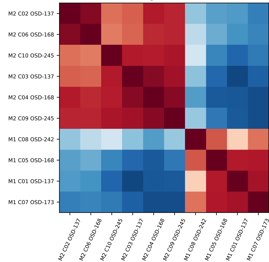
BridgeRNA512
