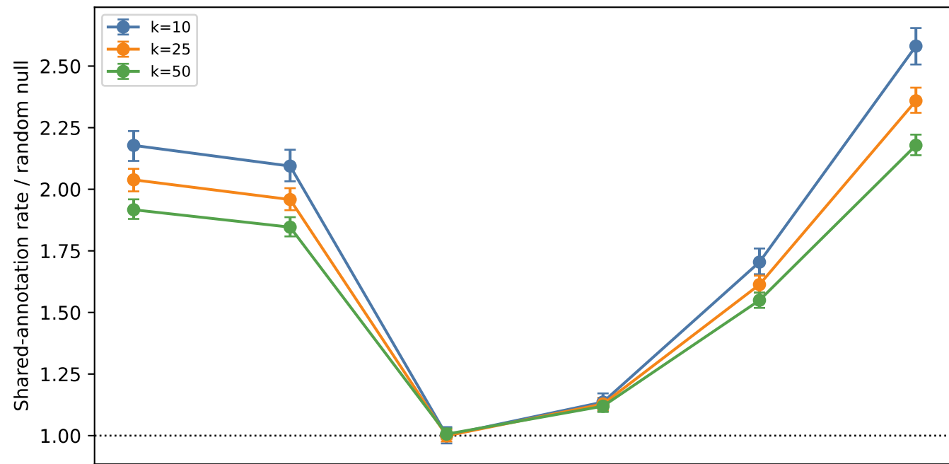
TCGA — GO
