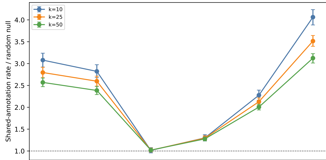
TCGA — KEGG
