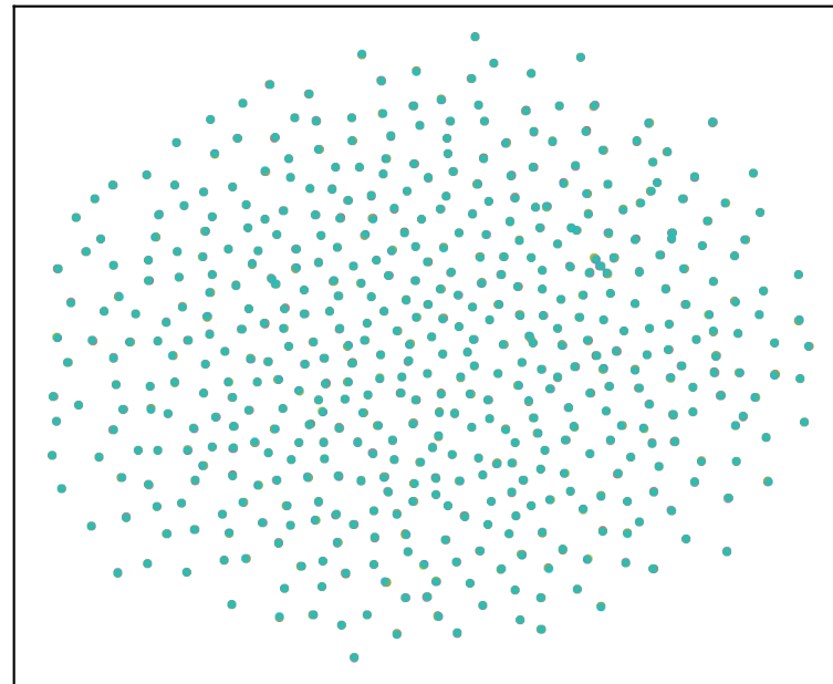
TCGA L6_middle UMAP
