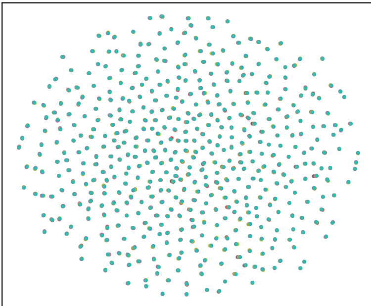
GTEx L6_middle t-SNE
