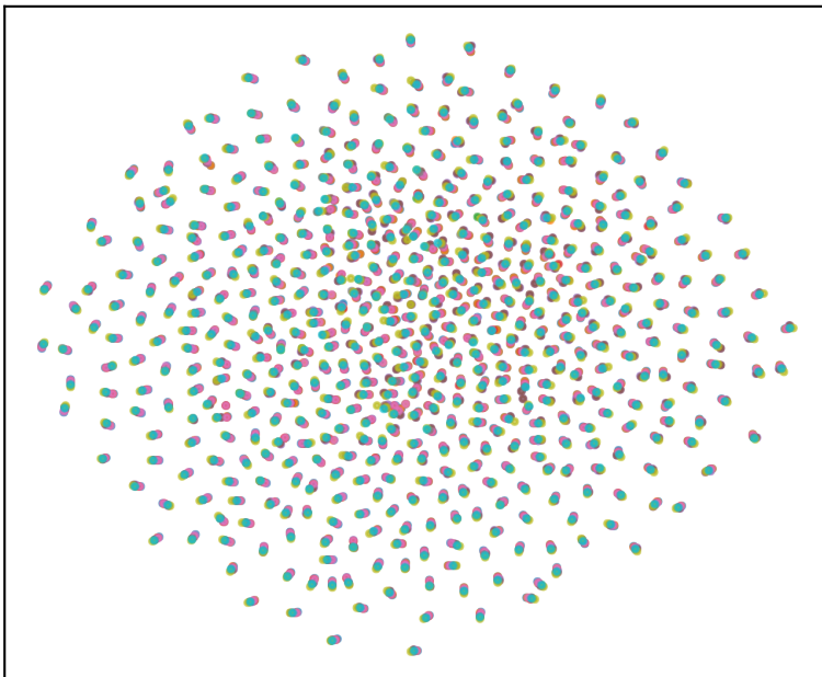
GTEx L12_final t-SNE
