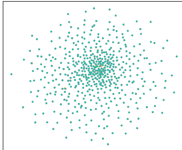
TCGA L12_final UMAP
