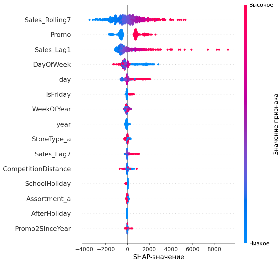
Рис. 4: Влияние признаков на прогноз XGBoost
