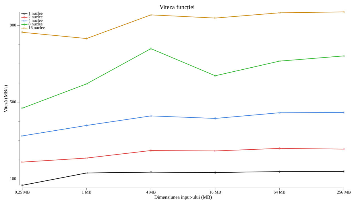
Figura 11: Viteza de procesare în funcție de dimensiunea datelor și de numărul de nuclee, pe procesorul AMD Ryzen 7 8845HS
