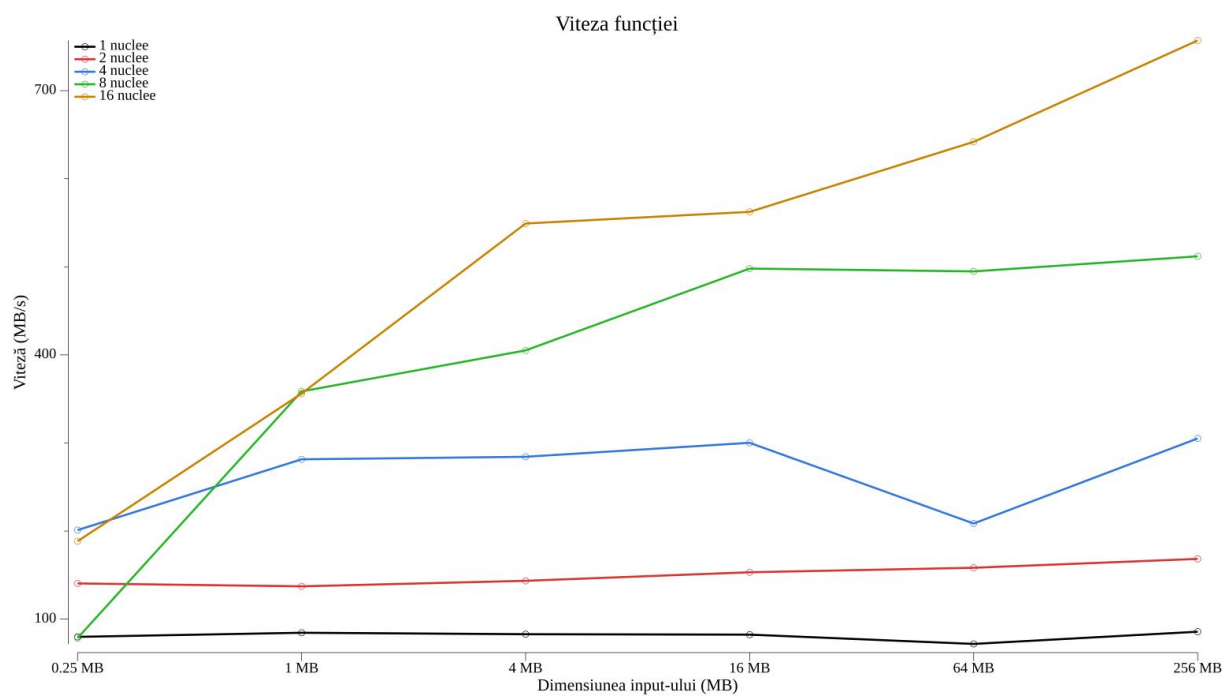
Figura 12: Viteza de procesare în funcție de dimensiunea datelor și de numărul de nuclee, pe procesorul Intel Xeon Platinum 8370C
