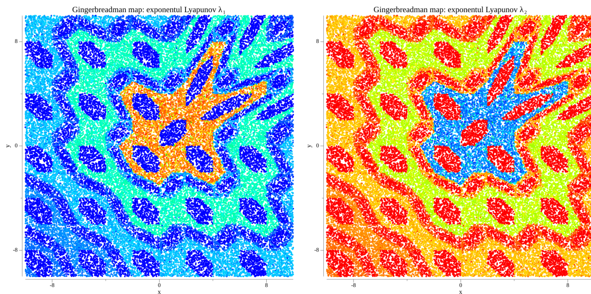
Figura 3: Exponenții Lyapunov \lambda_1 (stânga) și \lambda_2 (dreapta) ai gingerbreadman map
