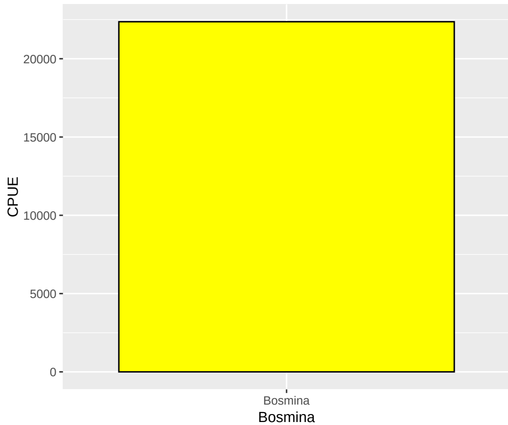
CPUE of Bosmina
