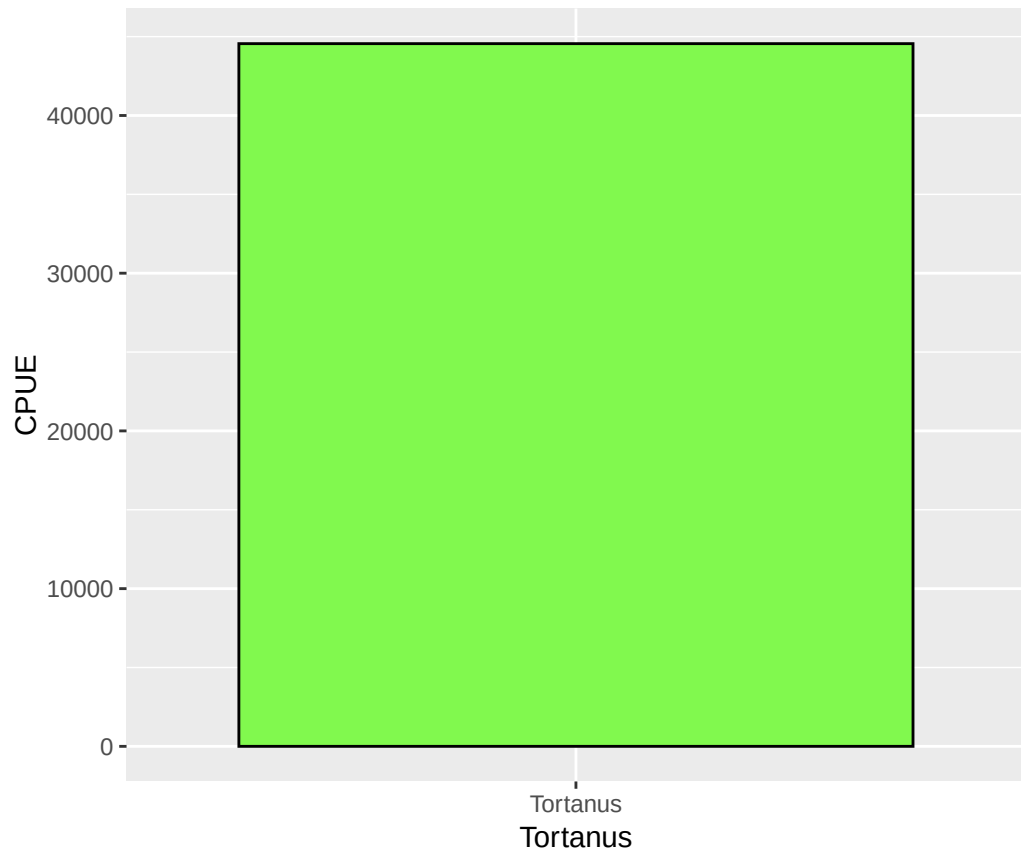
CPUE of Tortanus
