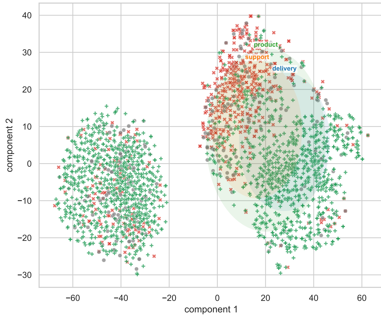
BERTimbau - t-SNE
