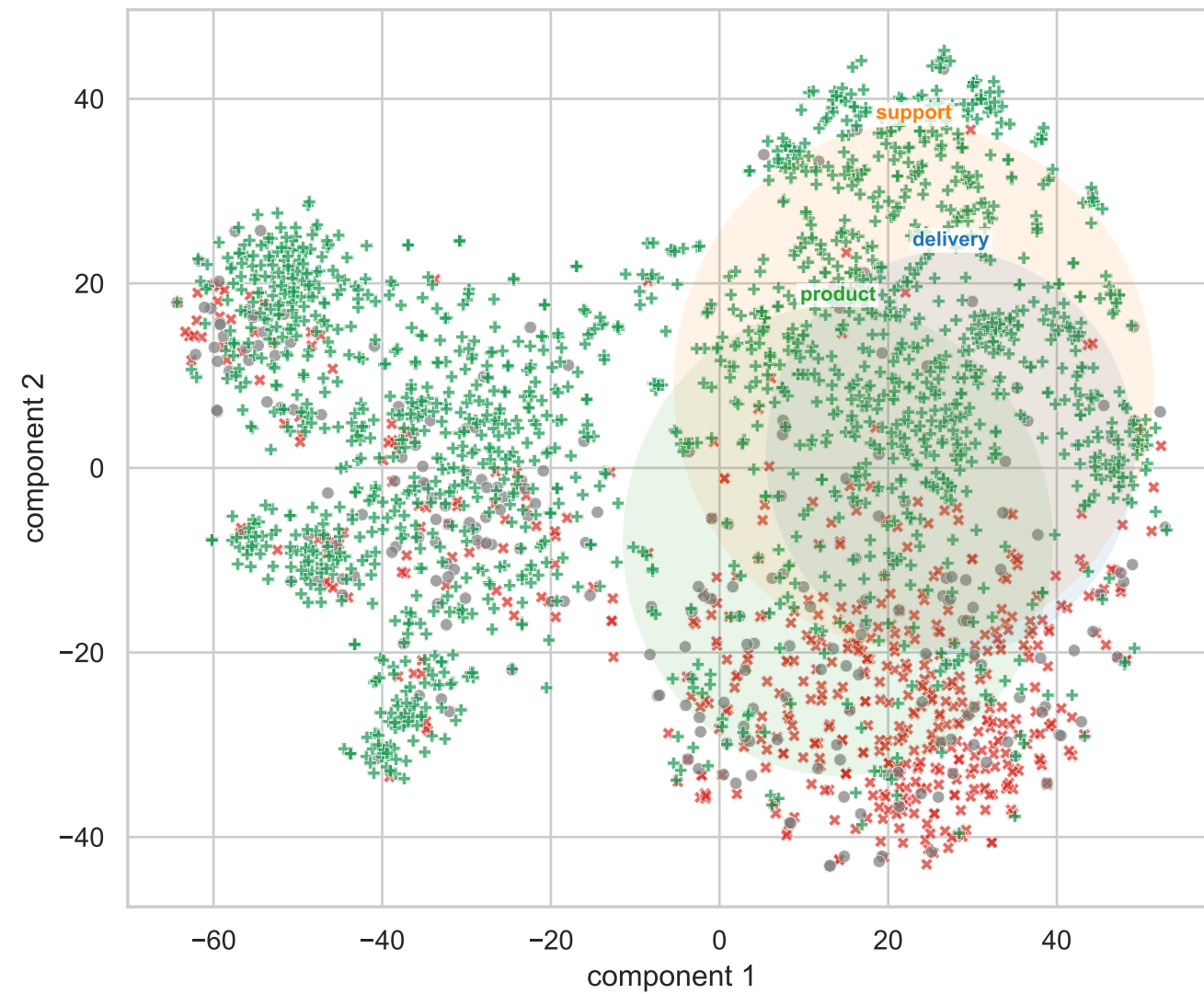
MiniLM - t-SNE
