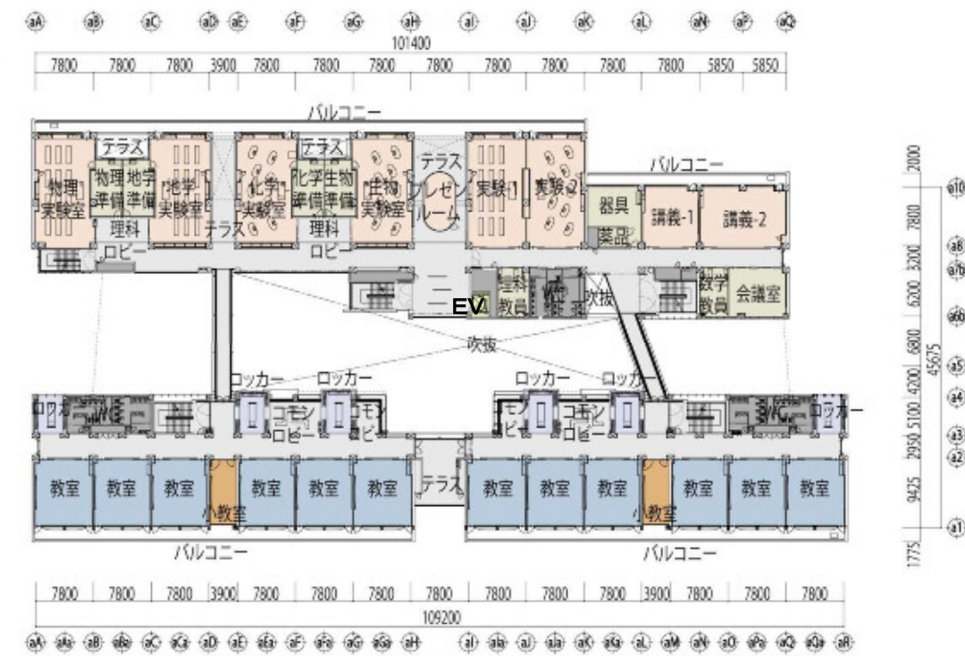
4階平面図
