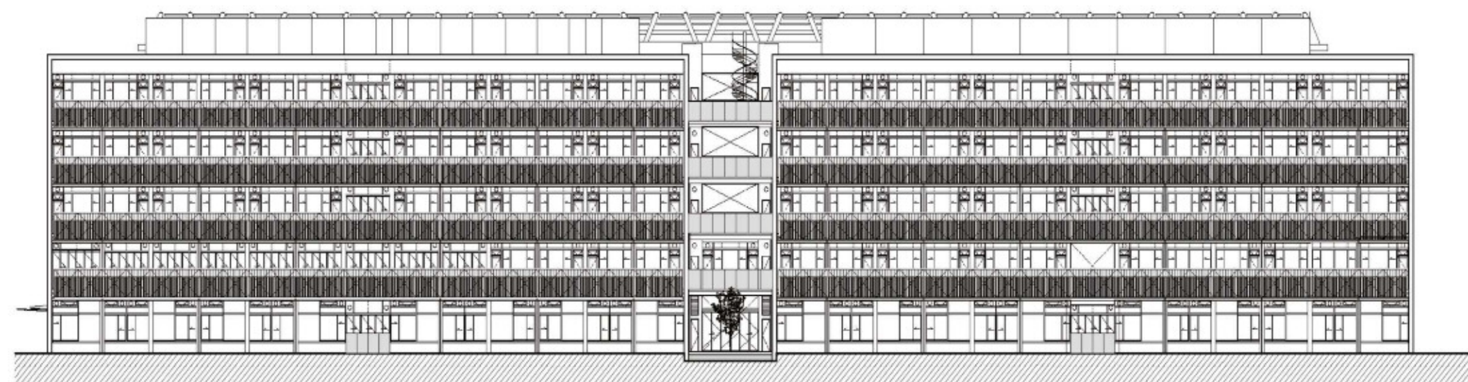
南立面図 校舎棟
