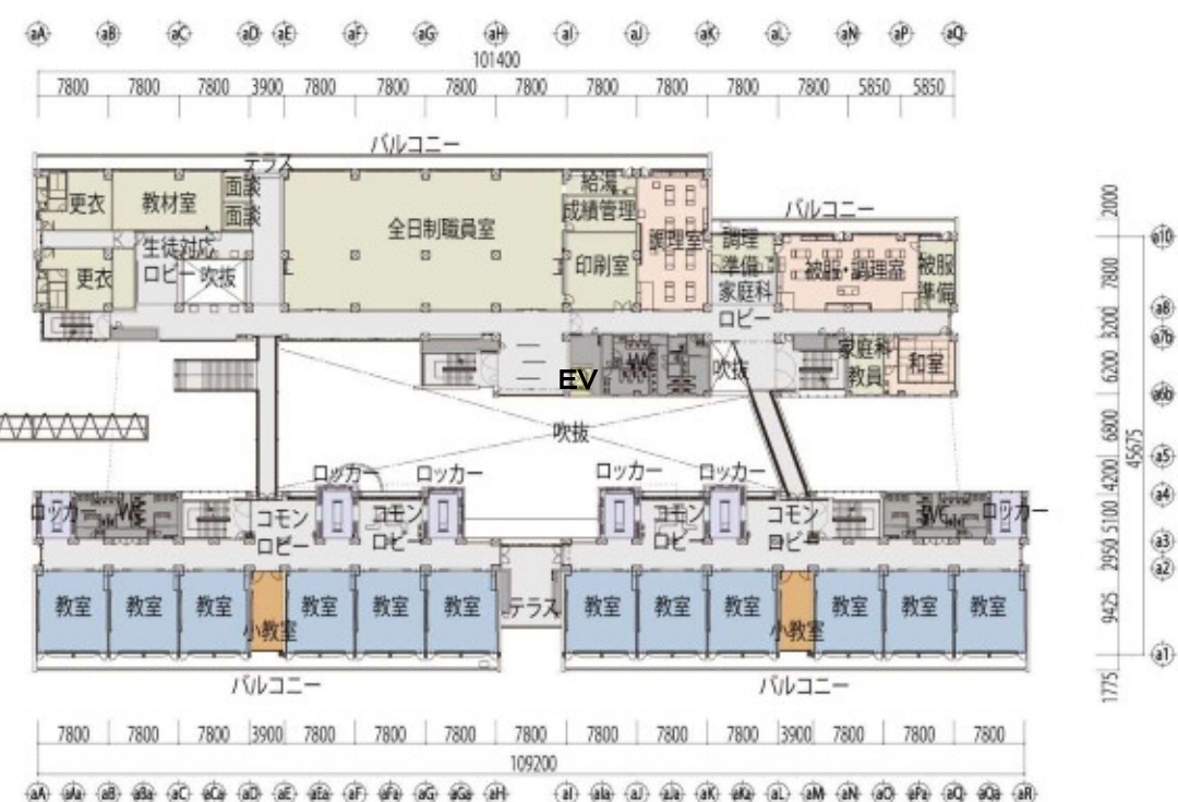
3階平面図
