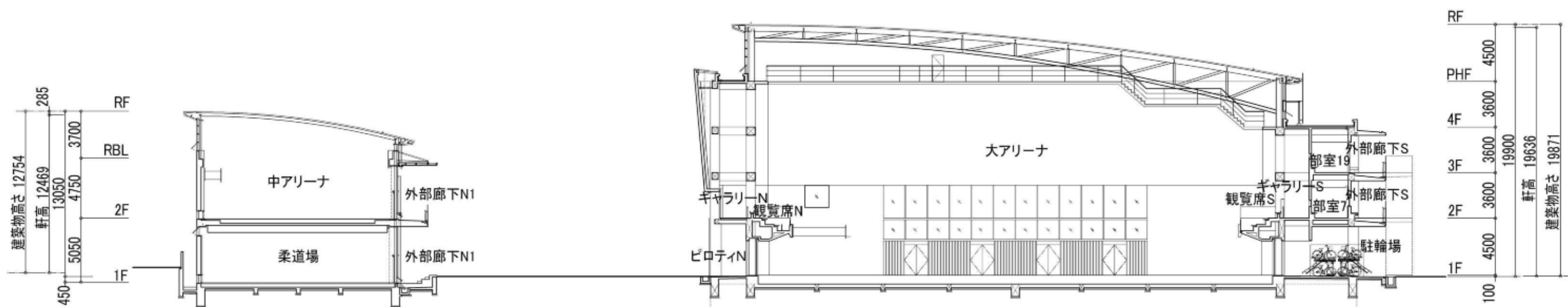
アリーナ棟断面図
