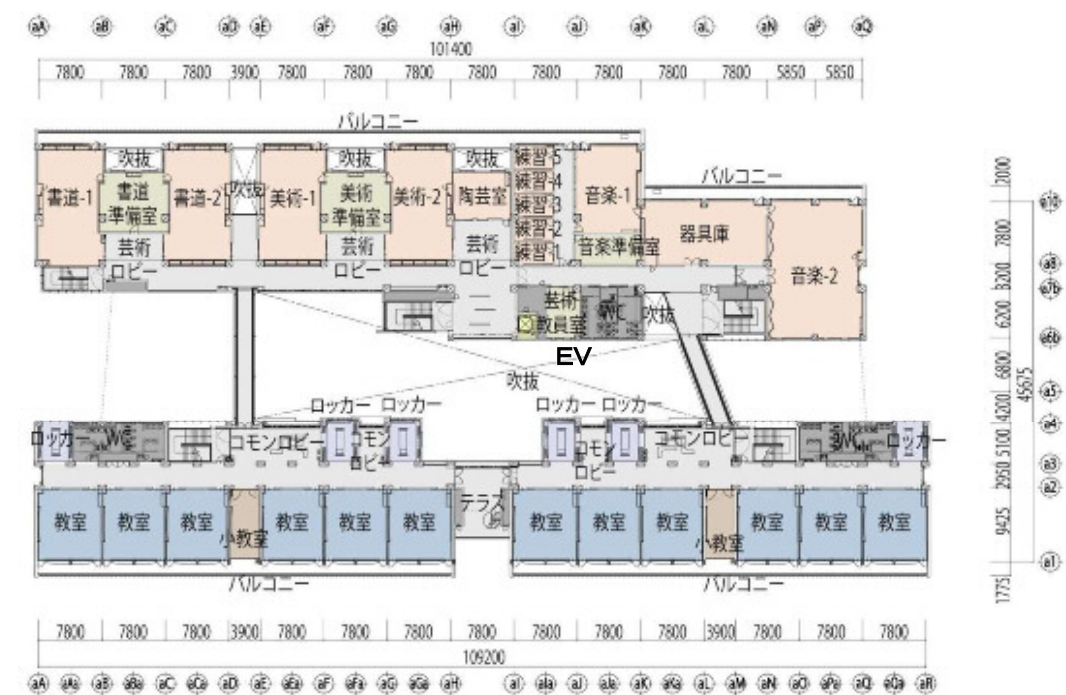
5階平面図
