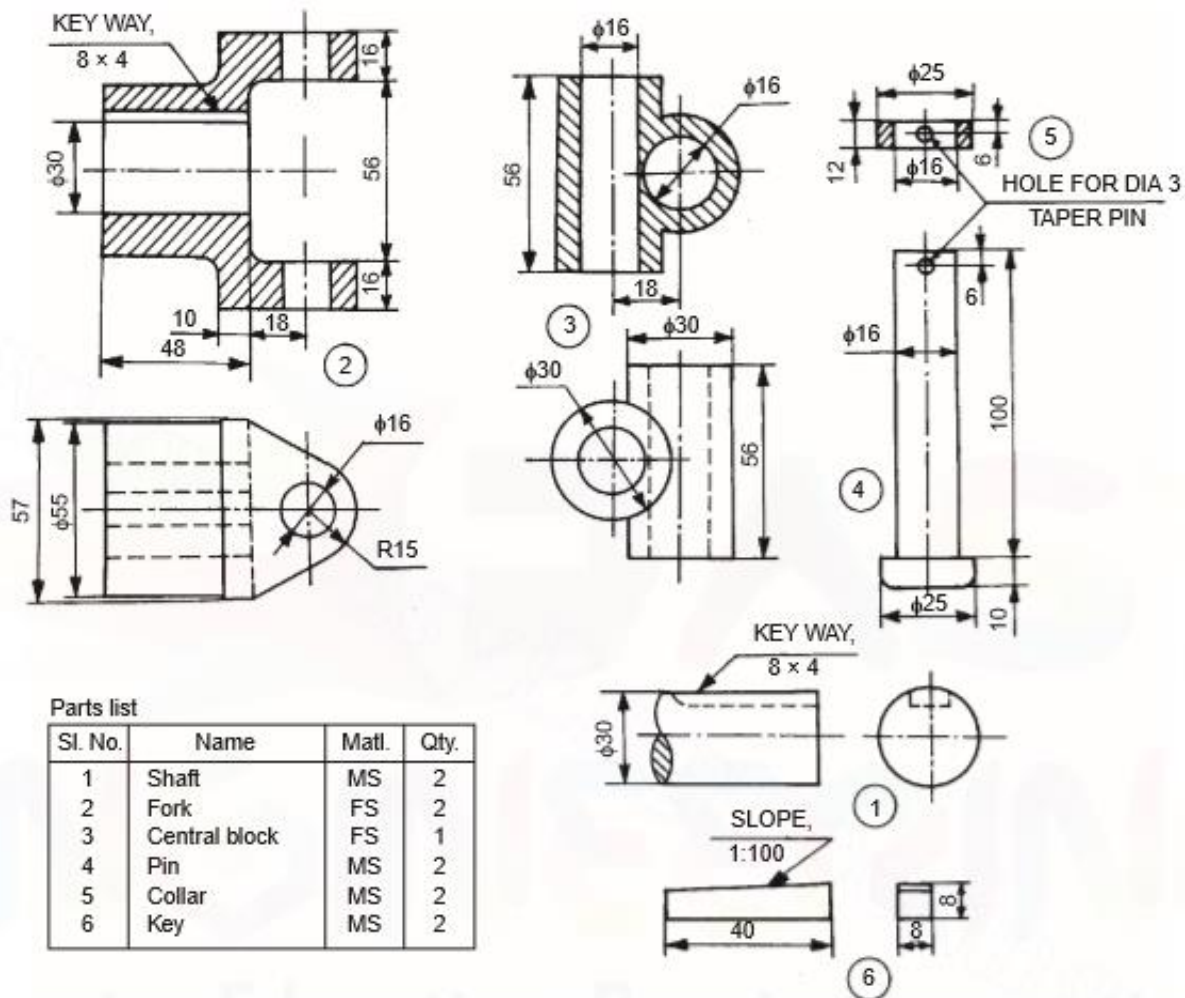
Fig. 18.44 Universal coupling
