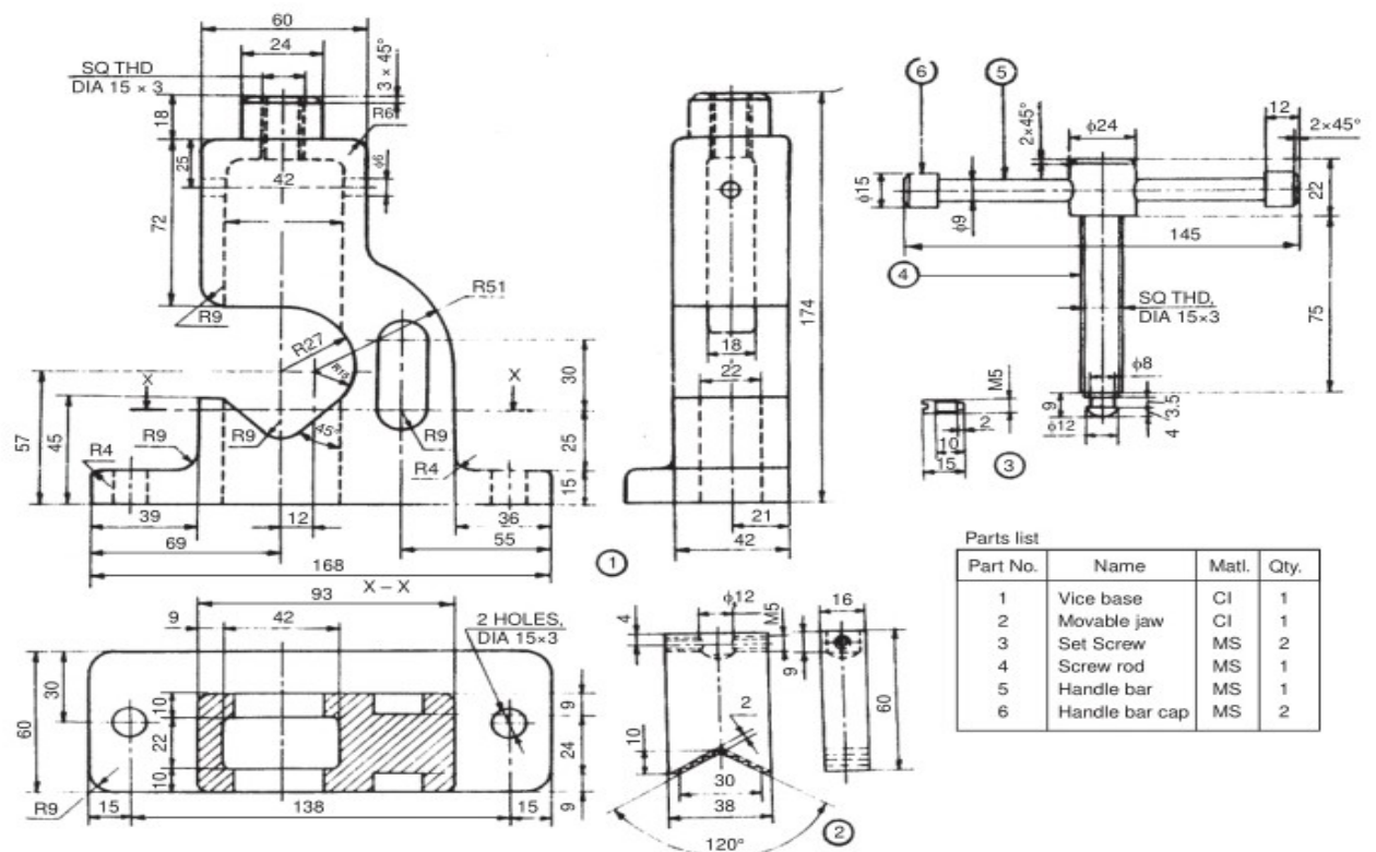
Fig. 18.52 Pipe vice
