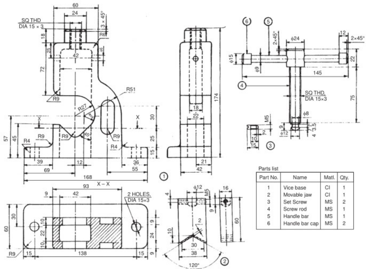
Fig. 18.52 Pipe vice
