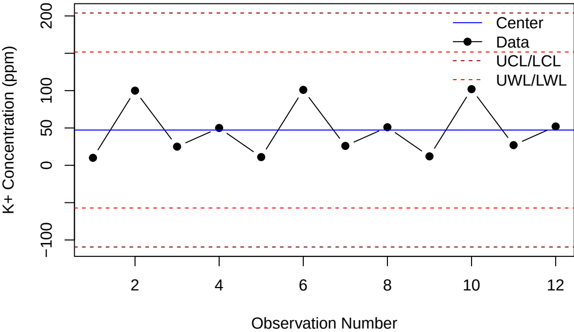
I-Chart
