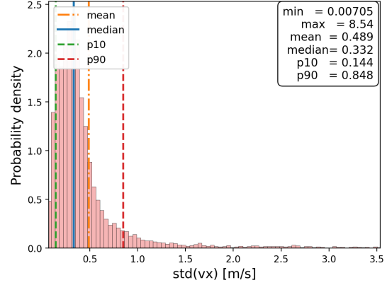
(d) Truck: variability of longitudinal velocity.
