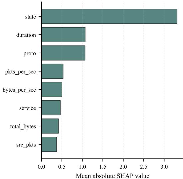
(b) ToN-IoT
