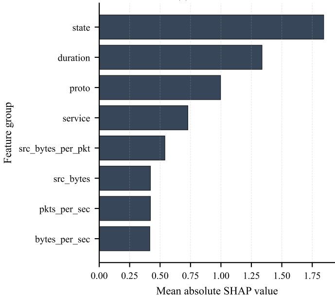
(a) UNSW-NB15
