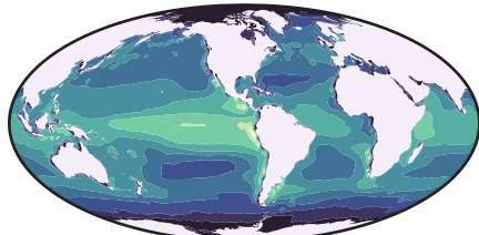
d. VGPM-Standard
