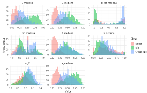
Histogramas por variable y clase
