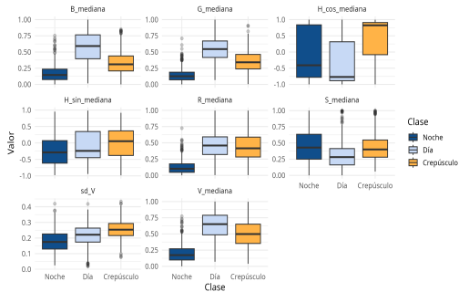
Distribución de variables (modelo base: RGB+HSV+sd(V))
