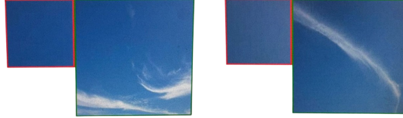
Figure 1: Imagen original vs Recorte en imágenes nubladas realmente despejadas
