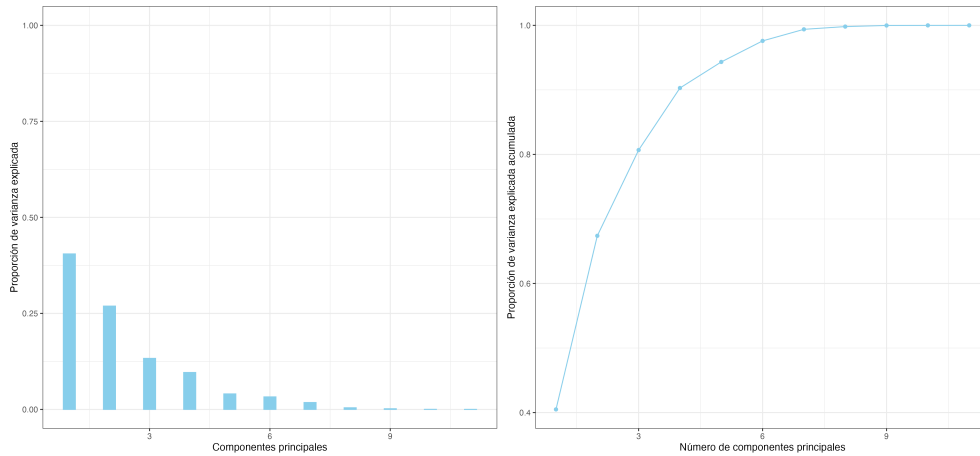
Figure 12: Proporciones y proporciones acumuladas de varianza explicada por el PCA
