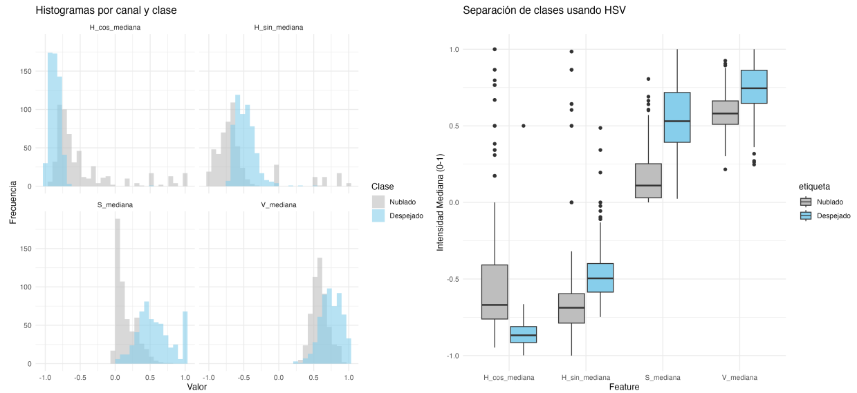
Figure 9: Histogramas y diagramas de caja de los canales HSV
